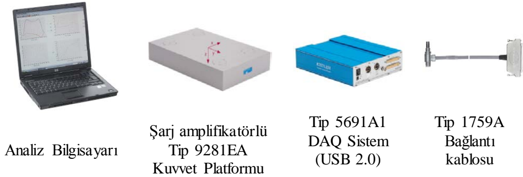
Şekil 41. Kuvvet Platformu Ölçüm Seti
