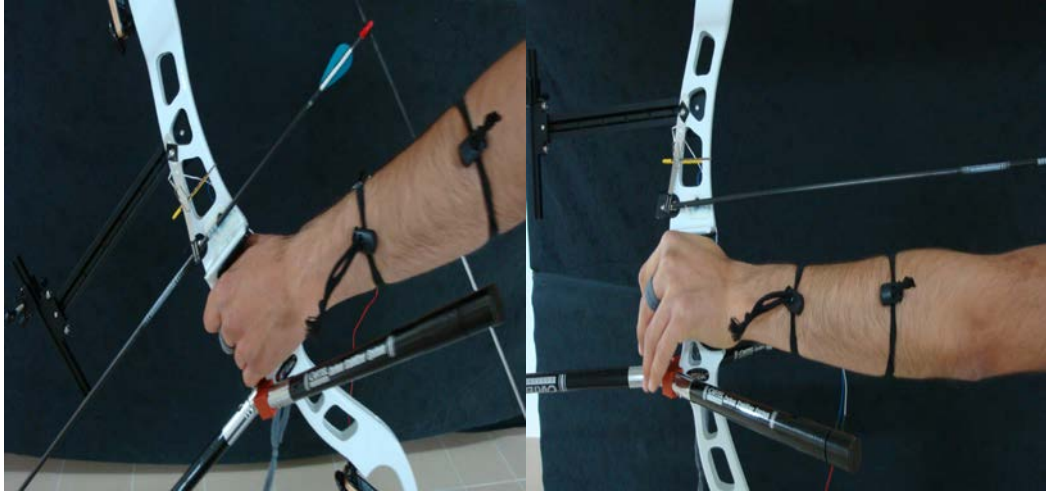
Şekil 46. Klikır ve Klikır'ın Altına Yerleştirilen Düzenek
