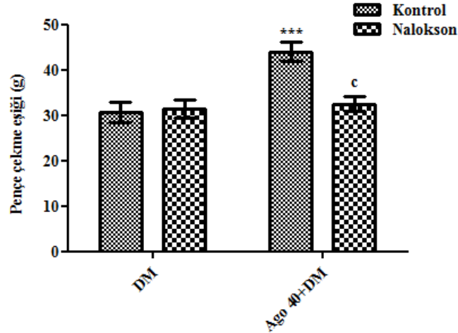
Şekil 13. Nalokson ( 1 \text{ mg.kg}^{-1} ) uygulamasının agomelatin ( 40 \text{ mg.kg}^{-1} ) ile indüklenen pençe çekme eşikleri üzerine etkisi. Serum Fizyolojik Uygulanan Diyabetik Kontrol Grubuna Göre Anlamli Farklılık ***p<0.001 , 40 \text{ mg.kg}^{-1} Agomelatin Uygulanan Diyabetik Grubuna Göre Anlamli Farklılık ^c p<0.001 , Çift Yönlü Varyans Analizi, Takiben Bonferroni Çoklu Karşılaştırma Testi, n=8 .
