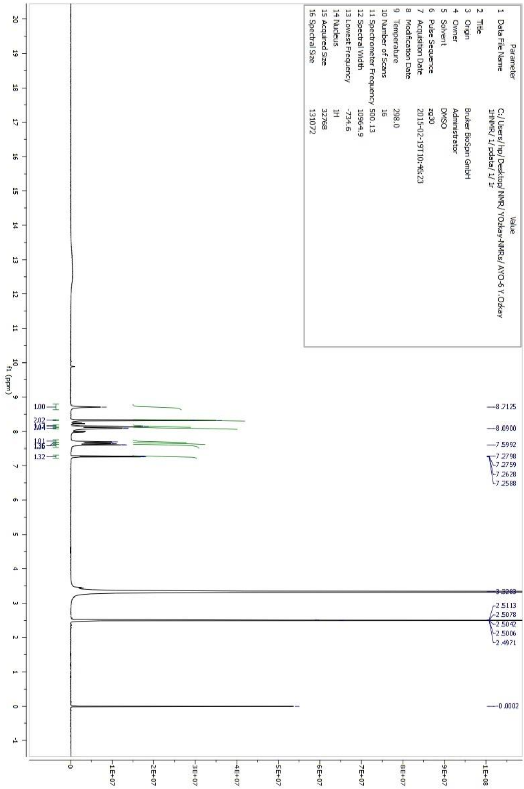
Şekil 85. Bileşik C6'ya Ait 1 H-NMR Spektrumu
