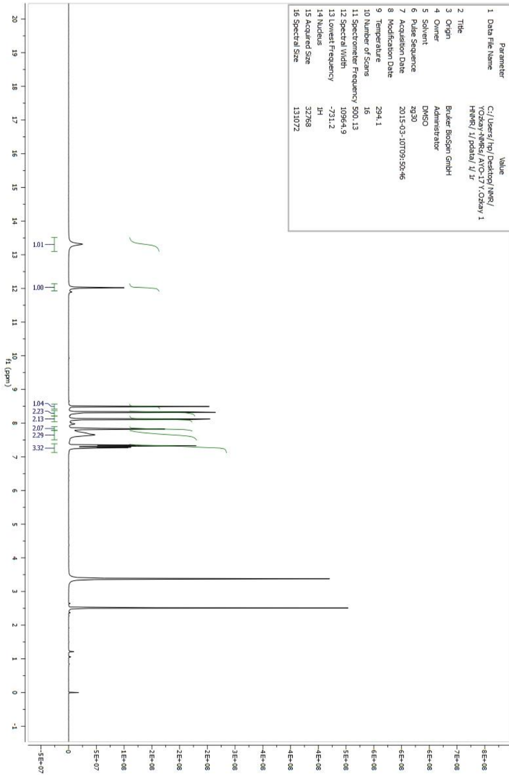
Şekil 129. Bileşik C17'ye Ait 1 H-NMR Spektrumu
