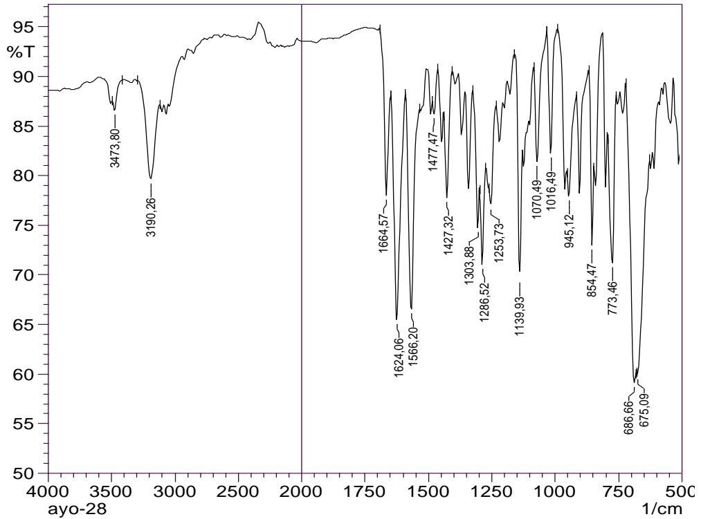
Şekil 168. Bileşik C27'ye Ait IR Spektrumu
