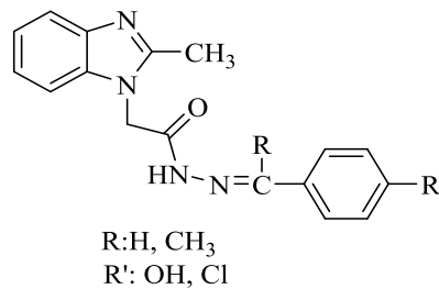
Şekil 48. N' -(Arilmetiliden)-2-(2-metil-1H-benzimidazol-1-il)asetohidrazitTürevi Bileşiklerin Kimyasal Yapısı
