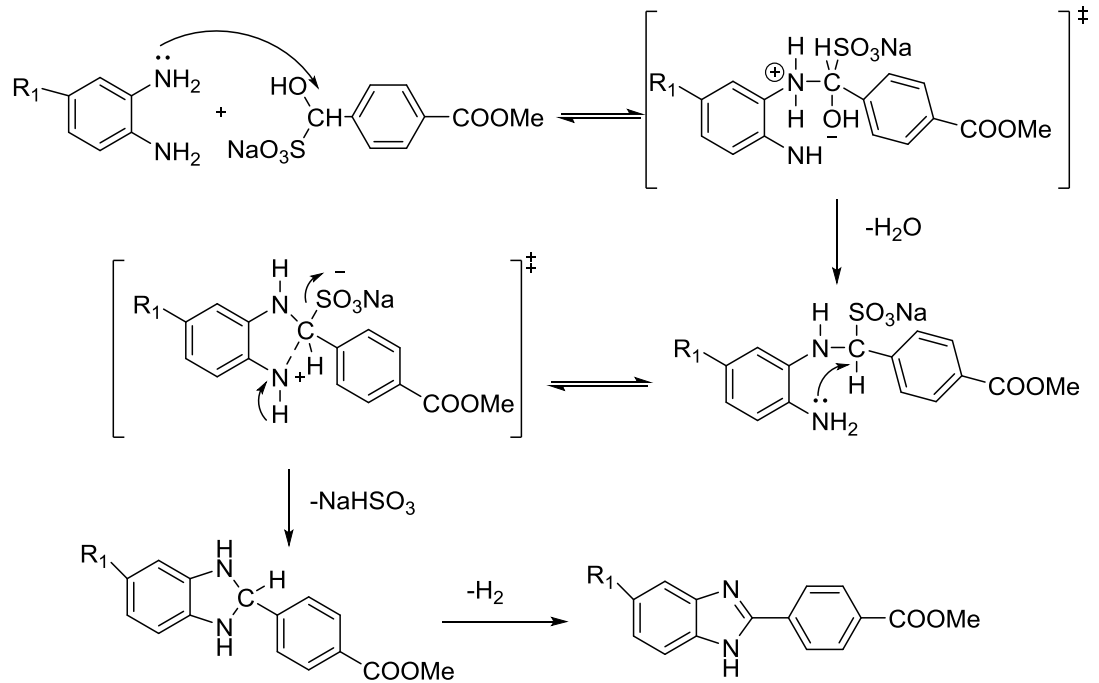
Şekil 62. Metil 4-(5(6)-Süstitüe-1H-Benzimidazol-2-il) Benzoat Türevlerinin Eldesi için Önerilen Reaksiyon Mekanizması
