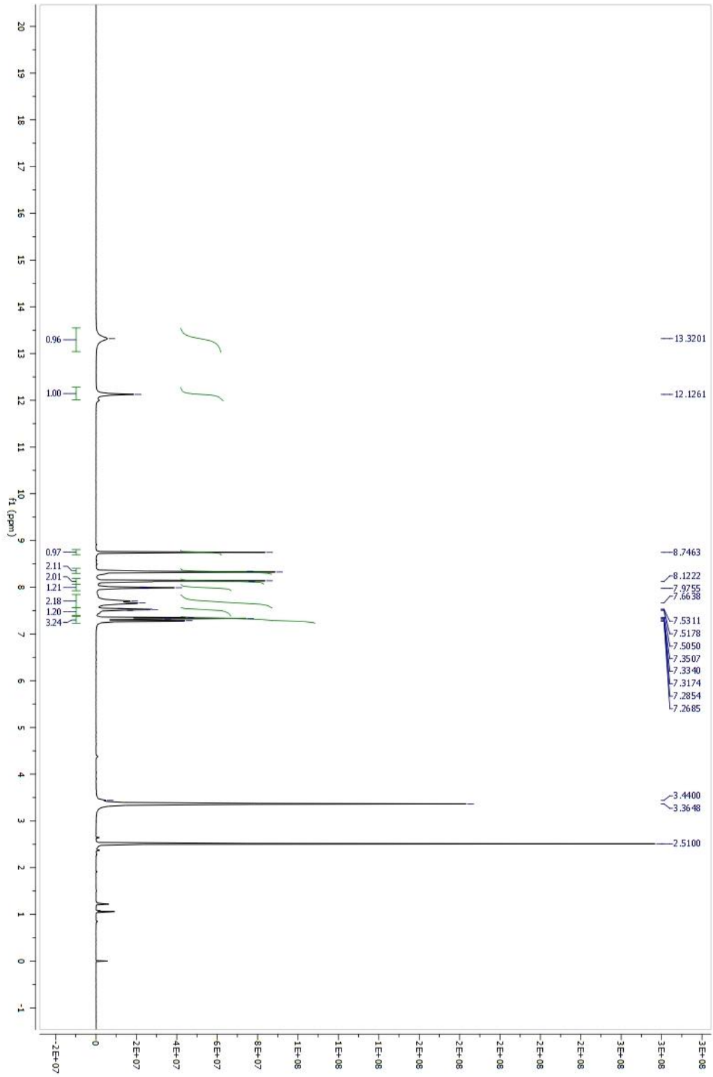
Şekil 121. Bileşik C15'e Ait ^1\text{H-NMR} Spektrumu
