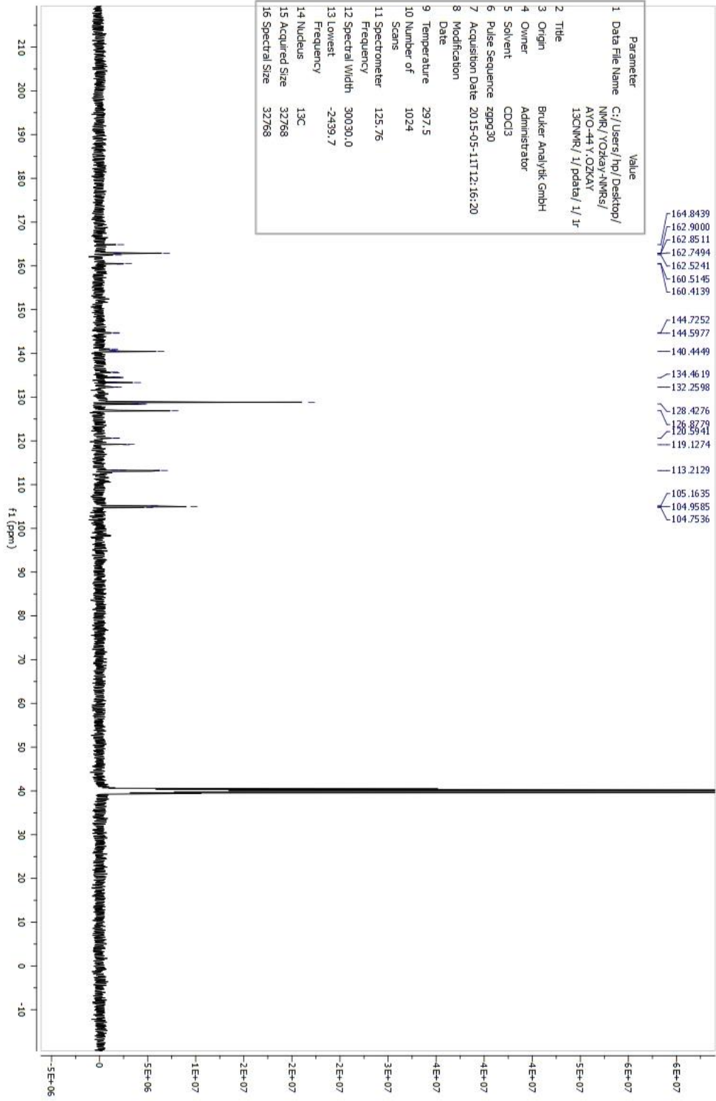
Şekil 234. Bileşik C43'e Ait 13 C-NMR Spektrumu
