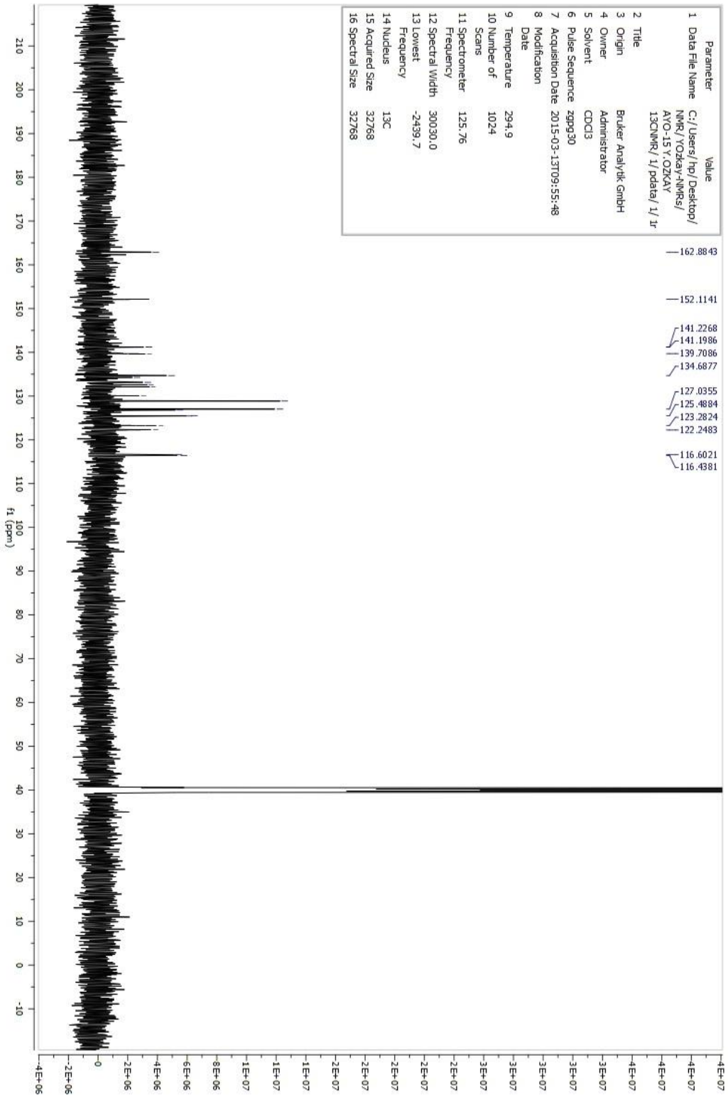
Şekil 122. Bileşik C15'e Ait ^{13}\text{C} -NMR Spektrumu
