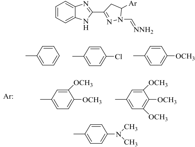
Şekil 42. 3-Benzimidazolil-5-aril-2-pirazolin-1-karboksaldehyt Hidrazon Türevi Bileşiklerin Kimyasal Yapısı
