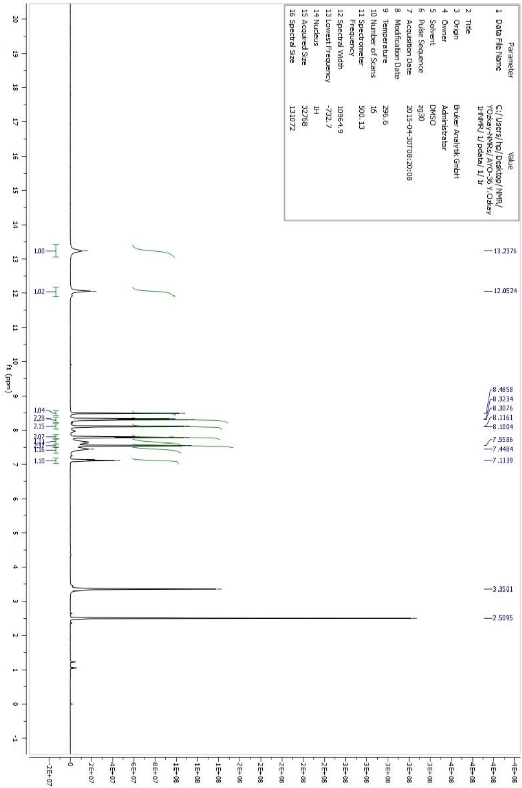
Şekil 201. Bileşik C35'e Ait ^1\text{H} -NMR Spektrumu
