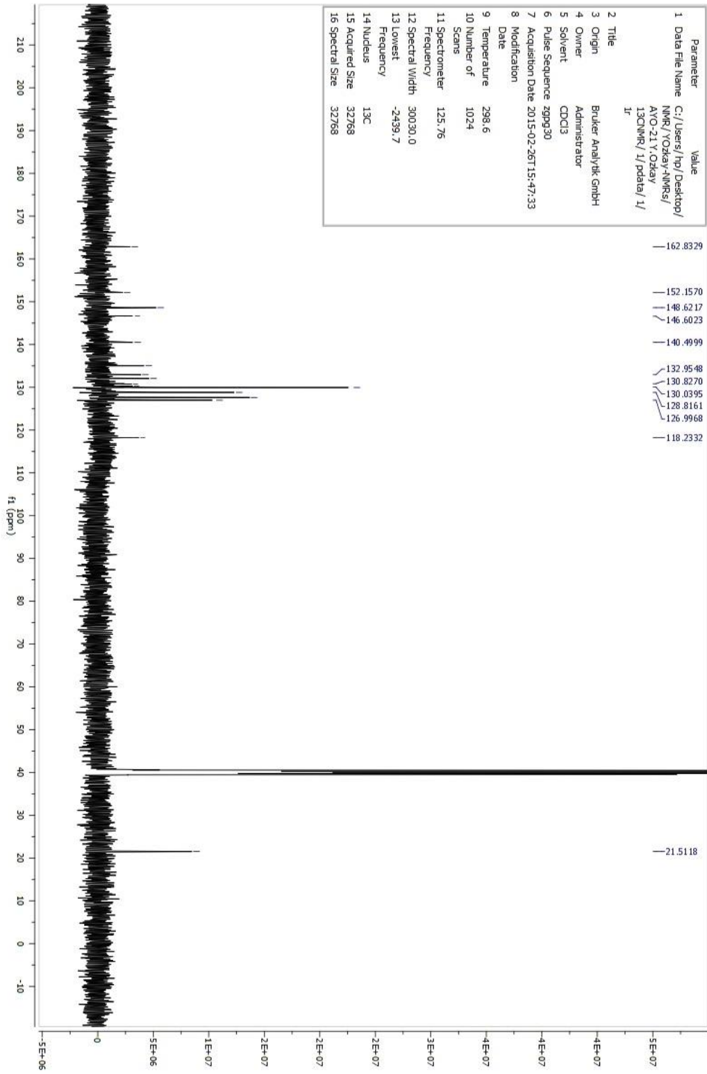
Şekil 146. Bileşik C21'e Ait 13 C-NMR Spektrumu
