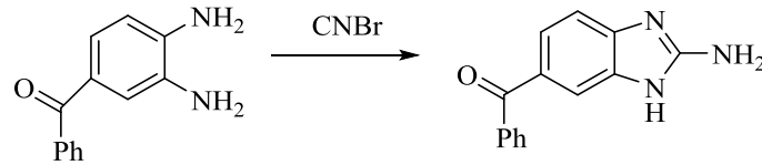
Şekil 28. o-Fenilendiaminin Bromosiyandır ile Reaksiyonuyla Benzimidazol Sentezi
