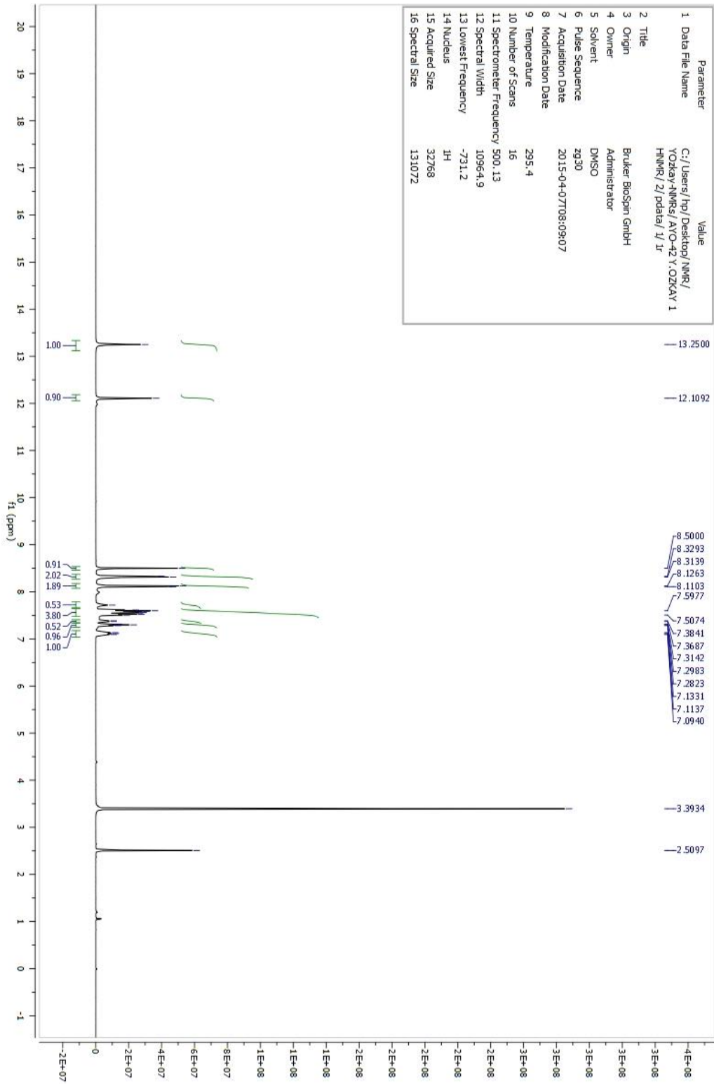
Şekil 225. Bileşik C41'e Ait 1 H-NMR Spektrumu
