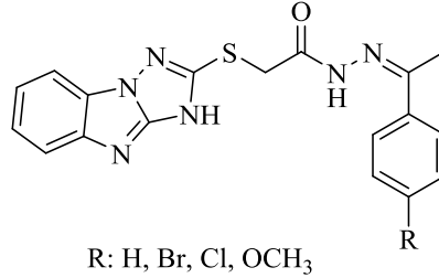
Şekil 49. N-( \alpha -ariletiliden)-2-(1H-1,2,4-triazol[2,3-a]benzimidazol-2-il sülfanil) asetohidrazit Türevi Bileşiklerinin Kimyasal Yapıları
