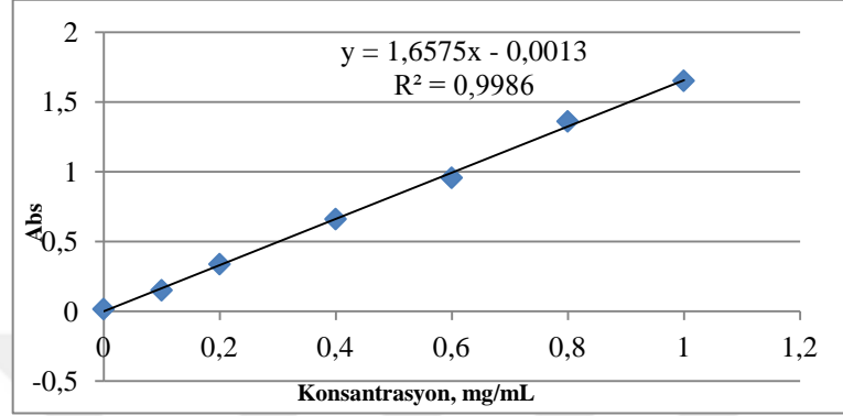
Şekil 27. Gallik Asit Lineer Eğrisi ve Hesaplama Denklemleri
