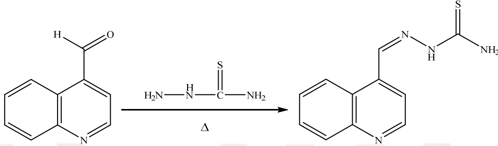
Şekil 27. 4-Kinolinkarboksaldehit tiyosemikarbazonun Sentezi
