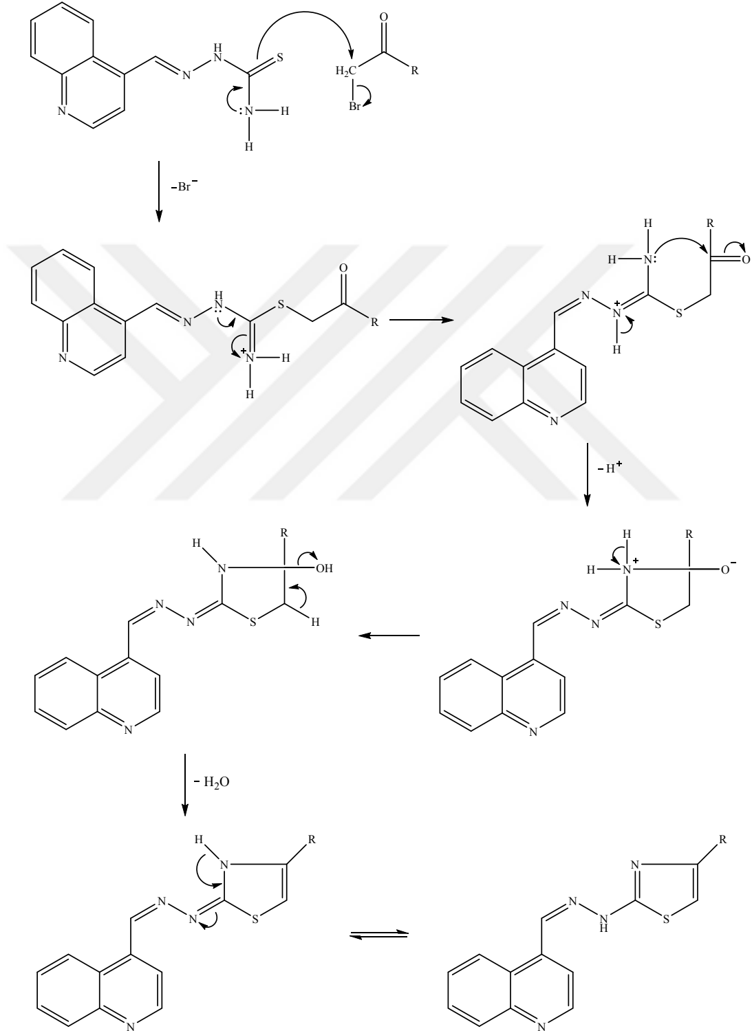
Şekil 30. Sonuç Bileşiklerinin Elde Edilişi için Önerilen Mekanizma
