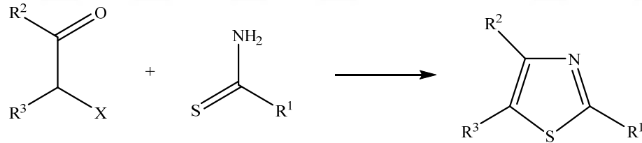
Şekil 9. \alpha -Haloketonların Tiyoamidler ile Reaksiyonu
