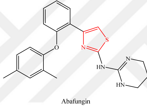
Şekil 1. Tiyazol Halka Yapısı Taşıyan Antifungal Etkili Ajanlar
