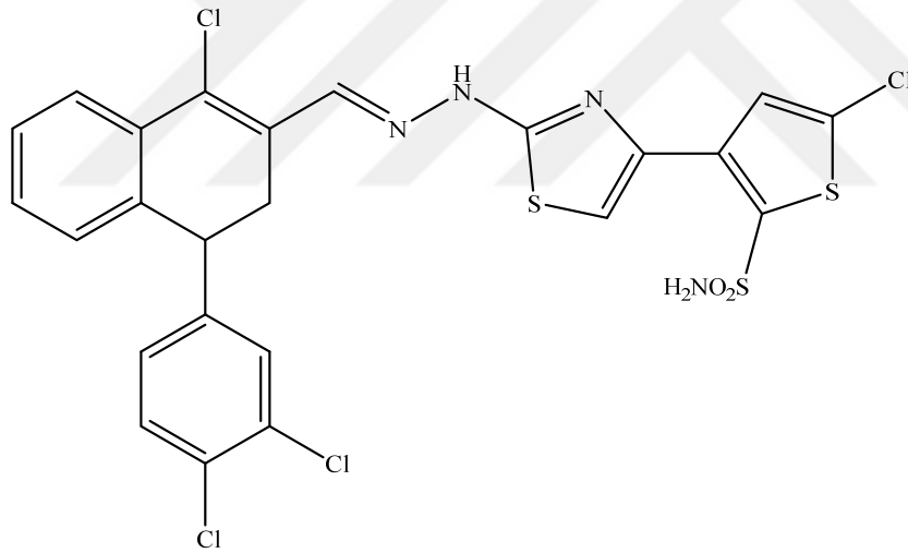
Şekil 23. 1-Kloro-4-(3,4-diklorofenil)-3,4-dihidronaftalen Halkası Taşıyan Tiyazol Türevleri
