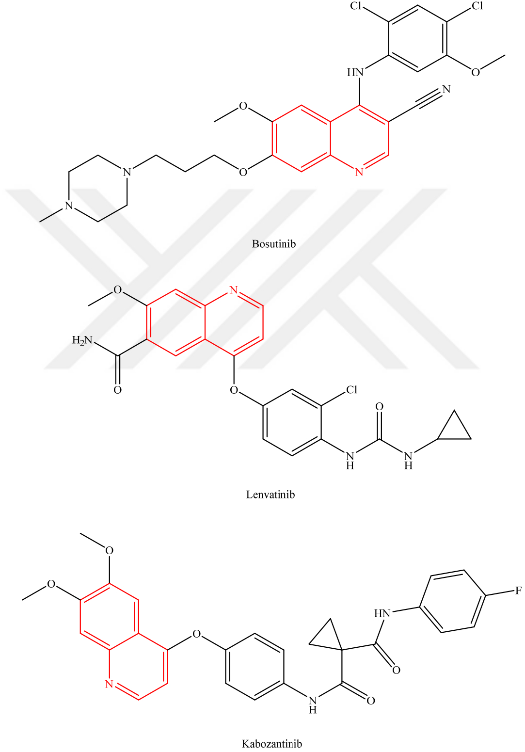
Şekil 4. Antikanser Etkili Kinolin Türevleri
