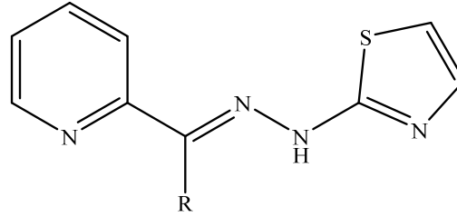
Şekil 14. Piridin Halkası Taşıyan Tiyazolil hidrazon Türevleri
