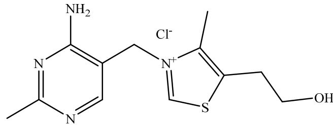
Şekil 6. Tiyamin
