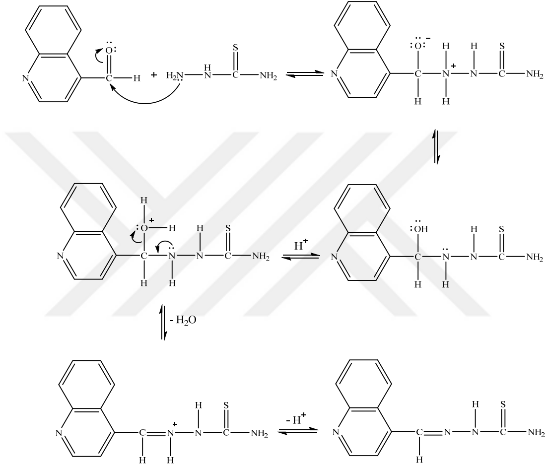
Şekil 29. 4-Kinolinkarboksaldehit tiyosemikarbazonun Elde Edilişi için Önerilen Mekanizma
