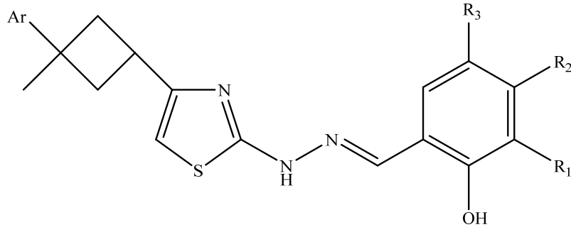
Şekil 15. 3-Süstitüe siklobütan Halkası Taşıyan Tiyazolil hidrazon Türevleri
