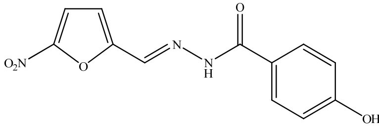
Şekil 12. Nifuroksazit
