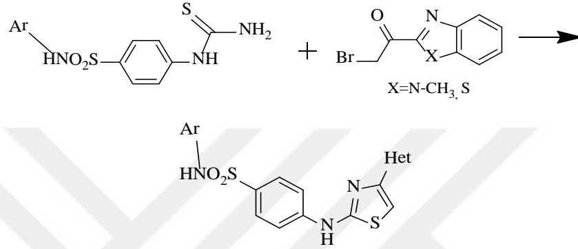
Şekil 4.9.4-[4-Süstitüetiiazol-2-il)amino]-N-arilbenzensülfonamit sentezi
