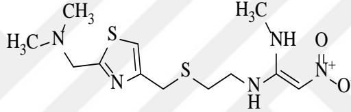
Şekil 2.28.Nizatidin molekülü
