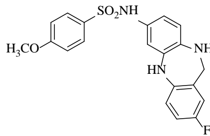
Şekil 2.16.ER-34410 molekülü
