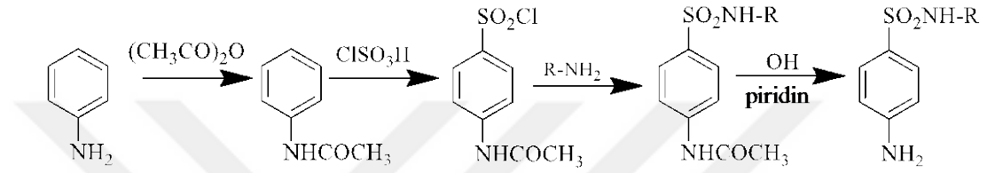
Şekil 2.5. Sülfonamitlerin aminlerden hareketle sentez yöntemleri
