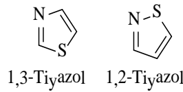
Şekil 2.18.1,3-Tiyazol ve 1,2-Tiyazol
