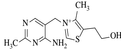
Şekil 2.33.Vitamin B1(tiyamin) molekülü
