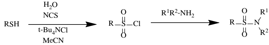
Şekil 2.8. Sülfonilamidlerin NCS ile sentez yöntemi
