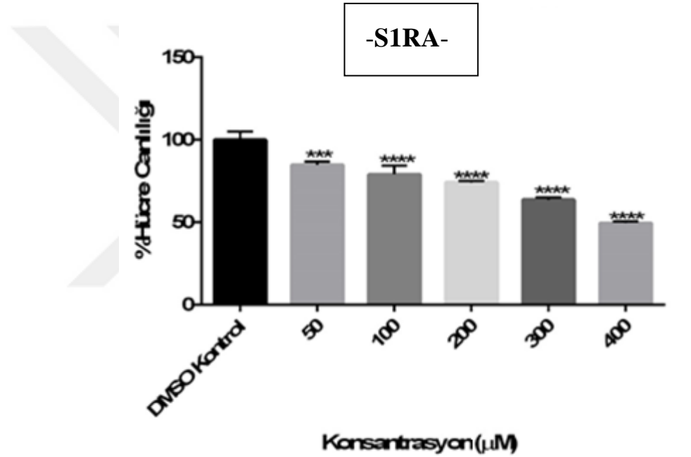
Şekil 5.1. U87MG hücrelerinde S1RA'nın 24.saatteki MTT testi sonuçlarına göre % hücre canlılığı oranları (Ortalama±Standart sapma, n=8, GraphPad Prism 6'da bulunan p değerleri; **** p<0,0001, ***p<0,001) Deneyler 3 bağımsız çalışma olarak tekrarlanmıştır, DMSO Kontrol: % 0,1 DMSO)
