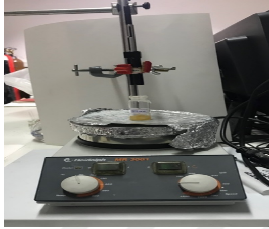
Görsel 3.1. KFME Deney Düzenegi
