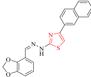
Şekil 5.55. Bileşik 2k
