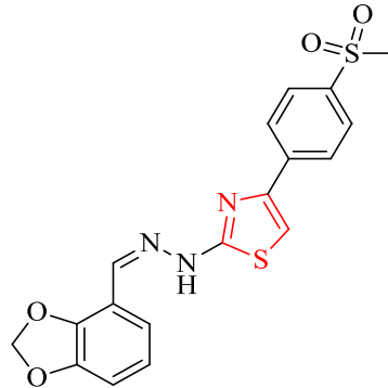
Şekil 5.50. Bileşik 2j
