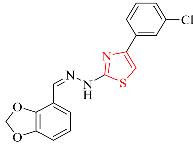
Şekil 5.65. Bileşik 2m
