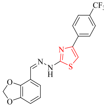
Şekil 5.20. Bileşik 2d
