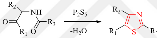
Şekil 2.7. Gabriel Sentezi
