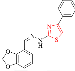
Şekil 5.5. Bileşik 2a
