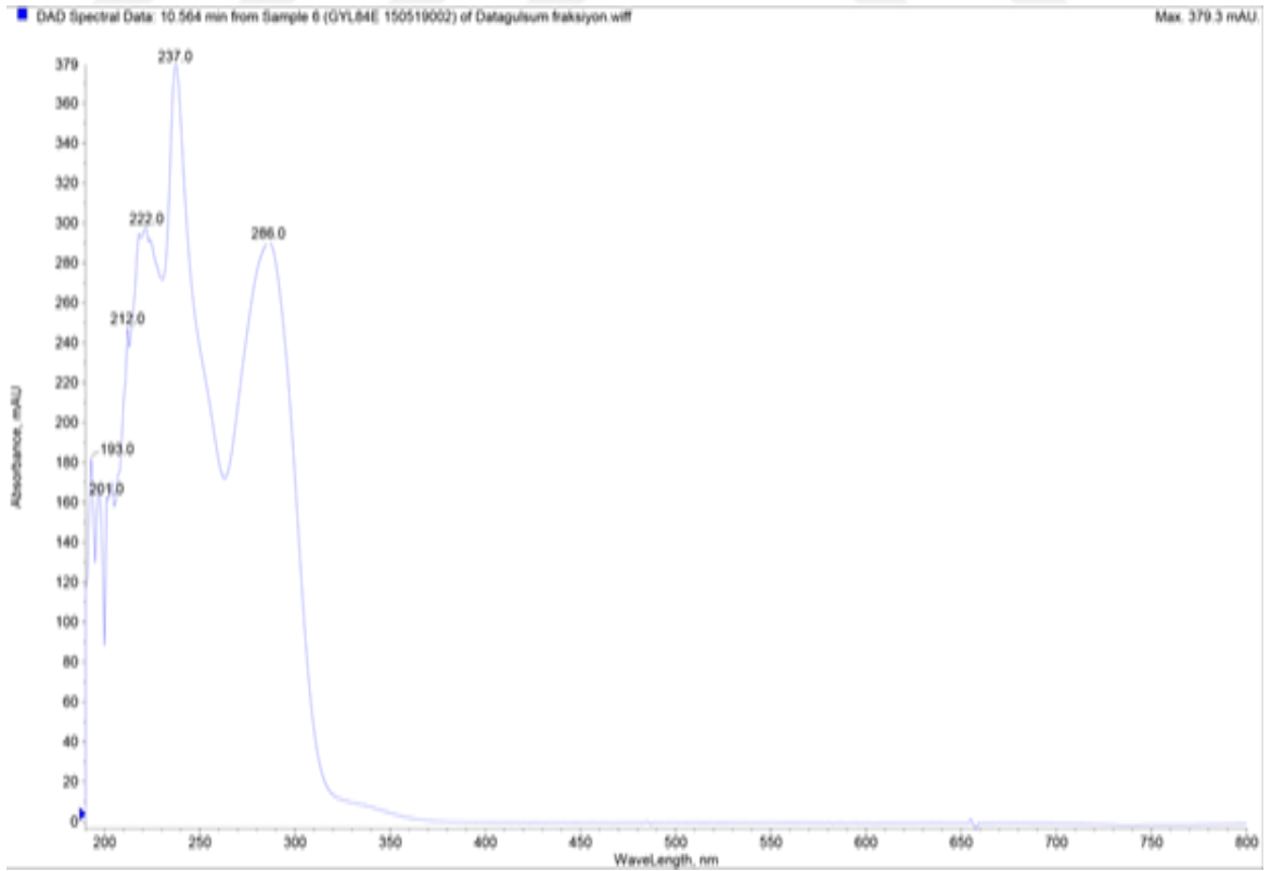
Şekil 4.48. Medioresinol/tuberonik asit heksoziti'ne ait UV spektrumu
