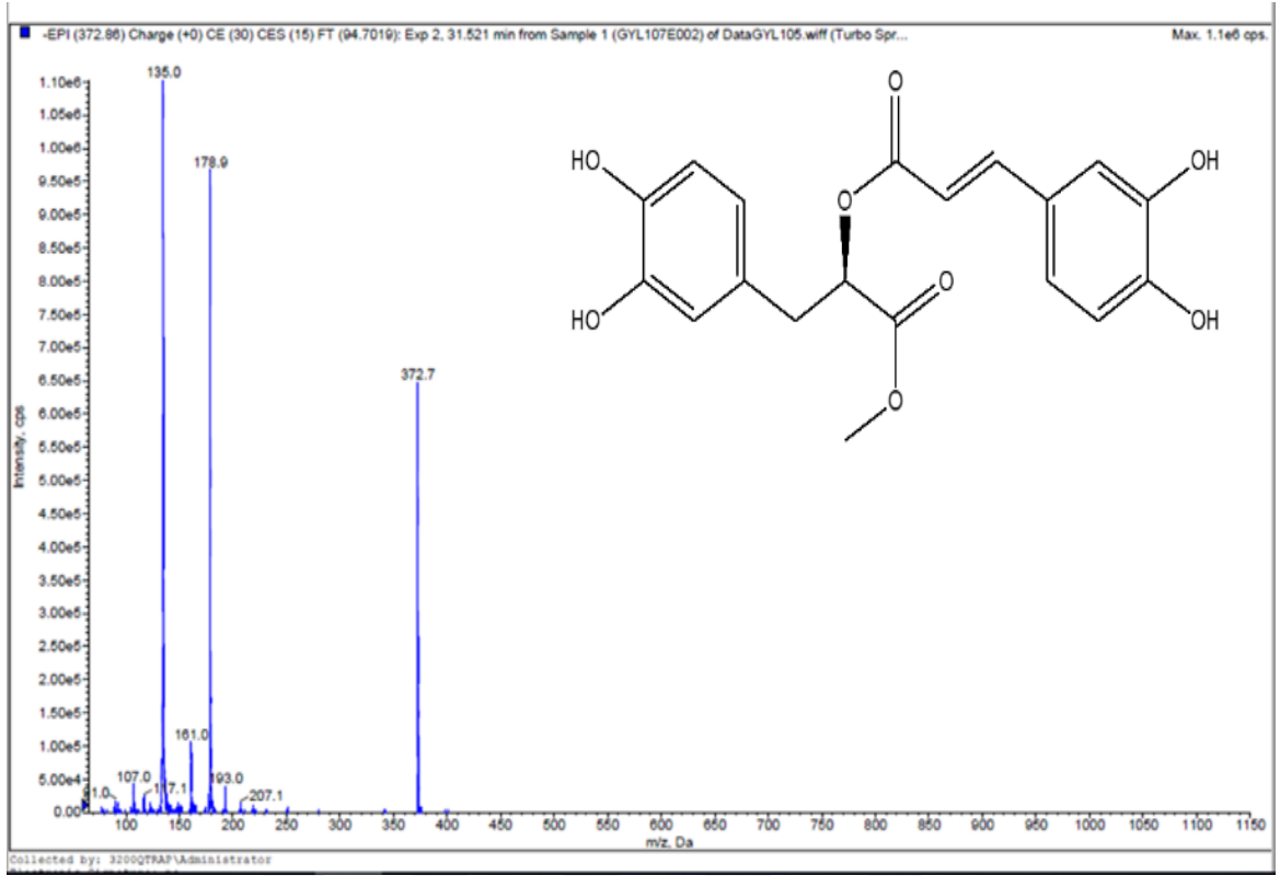
Şekil 4.8. Metil rozmarinat'a ait kütle spektrumu
