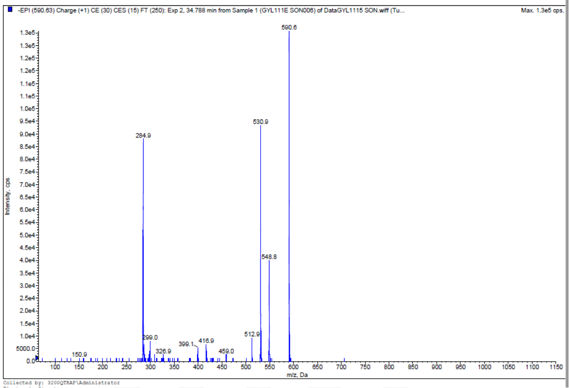
Şekil 4.33. Luteolin asetil dipentozit'e ait kütle spektrumu
