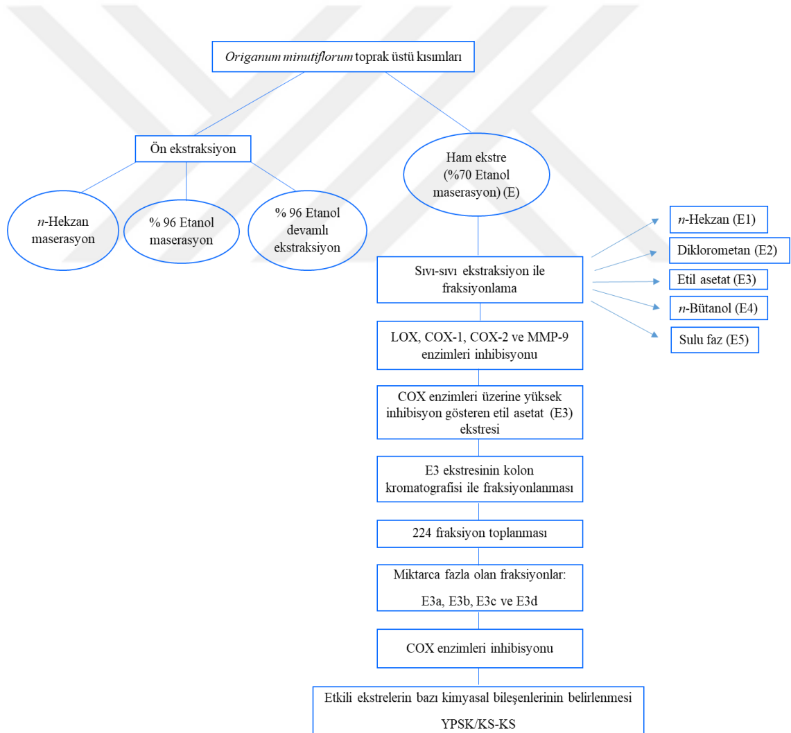
Şekil 3.1. Aktivite yönlendirmeli fraksiyonlama
