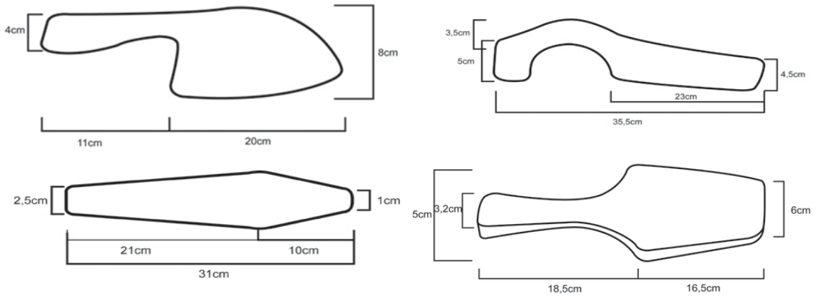
Şekil 31: Güney Kore’de Kullanılan Geleneksel Şekillendirme Aletleri, Çizimler: Roland Sipos.
