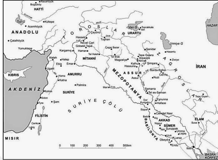
Şekil 3: Mezopotamya Haritası
