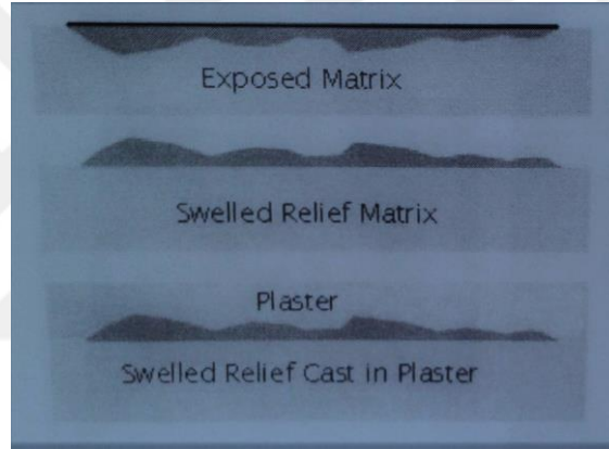
Resim-28 Şişirilmiş Jelatin Foto Rölyef Üretim Aşamaları
