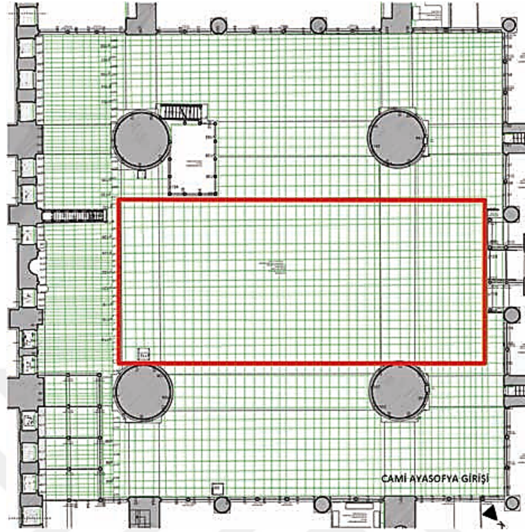
Şekil 14. Sultan Ahmed Camii içi jeoradar profillerinin oturumunu gösteren plan
