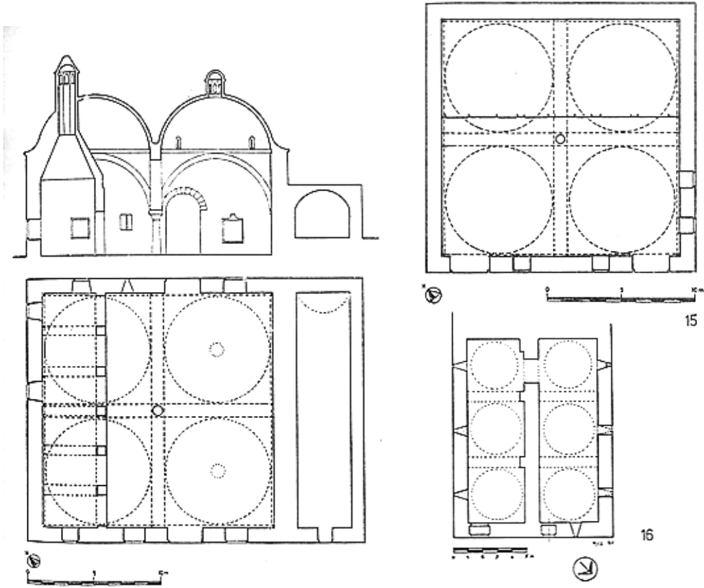
Şekil 21. Mutfak kesit ve planı, sağda fırın ve kilerin planı
