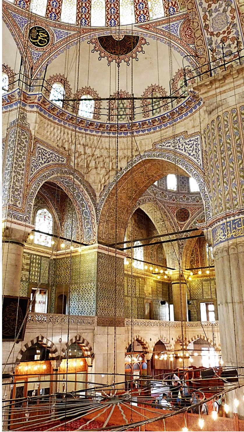
Resim 54. Harem-i enderûn batı duvarında kubbe, kemer, duvar ve pâye ilişkisi.
