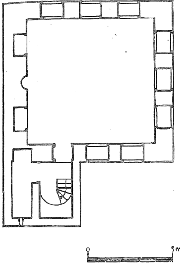
Şekil 23. Sultan Ahmed Külliyesi Sıbyan Mektebi Planı.
