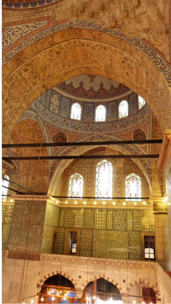
Resim 56. Sultan Ahmed Camii, kuzey cephesi ana giriş içeriden payanda ve mesnetleri.
