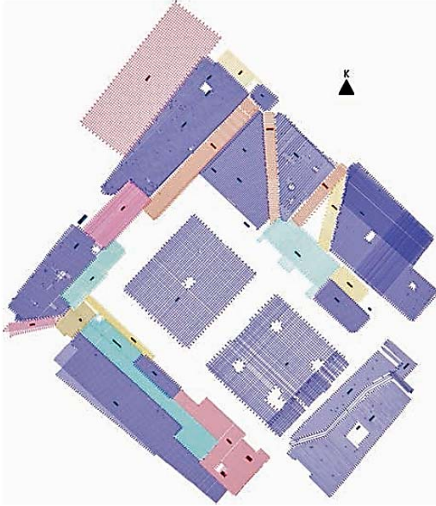
Şekil 12. Sultan Ahmed Camii'nden toplanan jeoradar tekniğiyle elde edilen profillerin derinlik ifadesi. Kaynak: Emre Evren ve komisyon, "Sultan Ahmet Camii'nde Arkeojeofizik Çalışmalar", Vakıf Restorasyon Yıllığı , S. IV, 2012, s.104.
