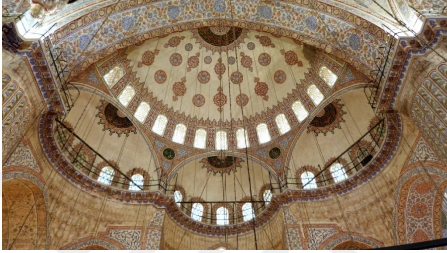
Resim 58. Sultan Ahmed Camii örtü sisteminde nîm kubbenin yükünü taşıyan tahfif (boşaltma) kemerleri.
