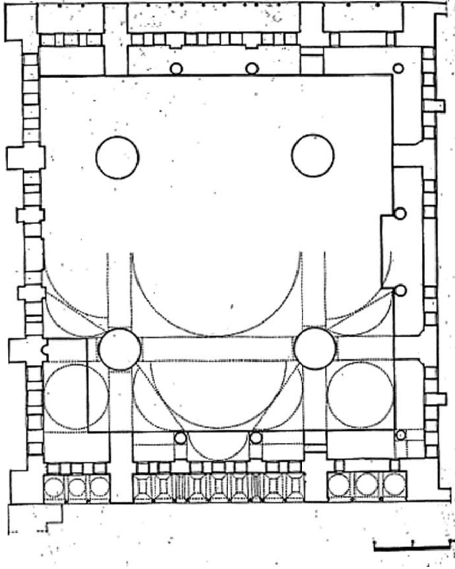
Şekil 5. Sultan Ahmed Camii harem-i enderun ve üst kat sofaların planı.
