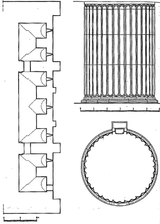
Şekil 10. Sultan Ahmed Camii bodrum kat ve şâh-pâye planı
