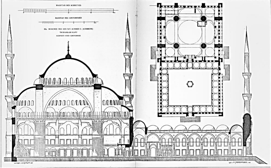
Şekil 4. Sultan Ahmed Camii, plan ve kesiti
