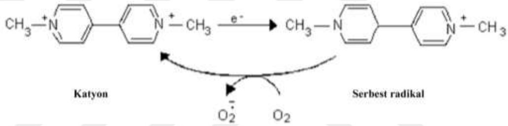
Şekil 2. 23. Paraquatın kimyasal yapısını ve ROT oluşumunu gösteren çizim (Bus ve Gibson, 1984).
