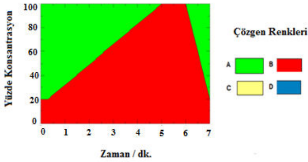
Şekil 4.3. Analizlerin yapıldığı, UHPLC-MS/MS cihazında hazırlanan gradyen programı. A% hareketli faz A'yı, B% hareketli faz B'yi göstermektedir
