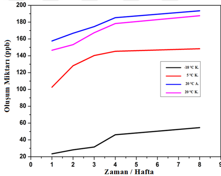
Şekil 4.14. Farklı sıcaklıktaki depolama koşullarında bekleme sonucu thiophanate-metil pestisitinden metaboliti olan carbendazim'in oluşum eğrisi
