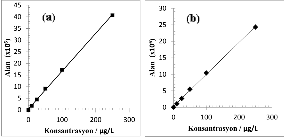
Şekil.4.7. a) Pirimicarb ve b) Aldicarb pestisitlerine ait kalibrasyon eğrileri
