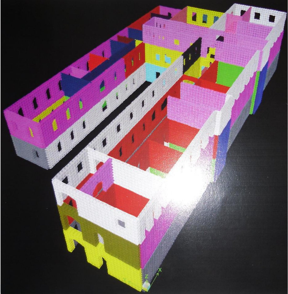
Ek-B.2: Cağaloğlu Anadolu Lisesi Eski Binanın 3D Boyutlu Modeli (Mevcut Durum Değerlendirme & Güçlendirme Projesi Öneri Raporu)
