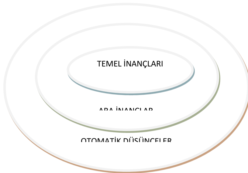
Şekil 2: Bilişsel Yapı
