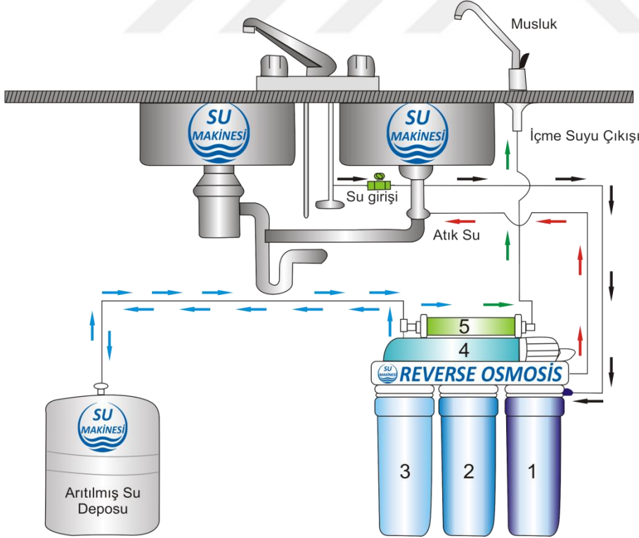
Şekil 2.8. Ev tipi ters osmoz akım şeması
