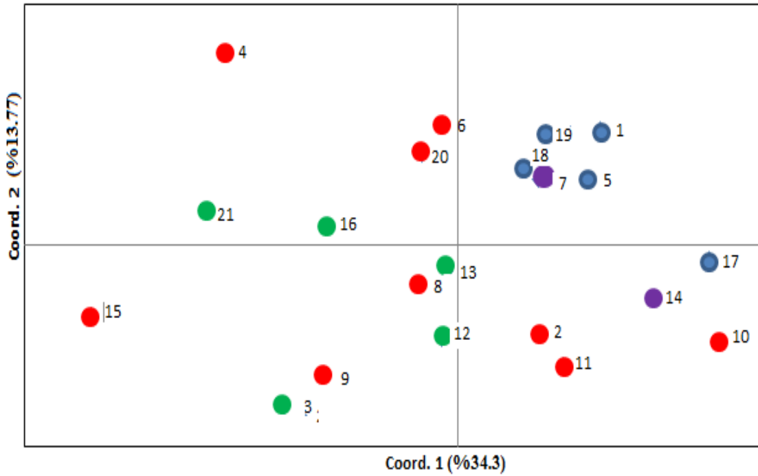
Şekil 4.8. ITAP'ların Nei (1972)'ye göre hesaplanmış genetik uzaklık değerleri kullanılarak yapılan PCoA sonucu (1. Adana-Pozantı, 2. Afyon-Sandıklı, 3. Ankara-Beypazarı, 4. Antalya-Elmalı, 5. Antalya-Gündoğmuş, 6. Antalya-Termessos 7. J. foetidissima , 8. Aydın-Efeler, 9. Burdur-Bucak, 10. Denizli-Acıpayam, 11. Denizli-Beyağaç, 12. Eskişehir-Mihalıççık, 13. Eskişehir-Seyitgazi, 14. J. polycarpus , 15. Isparta-Senirkent, 16. Karabük-Eskipazar, 17. Konya-Hadim, 18. Mersin-Mut, 19. Mersin-Tarsus, 20. Muğla-Seydikemer, 21. Sinop-Boyabat)
