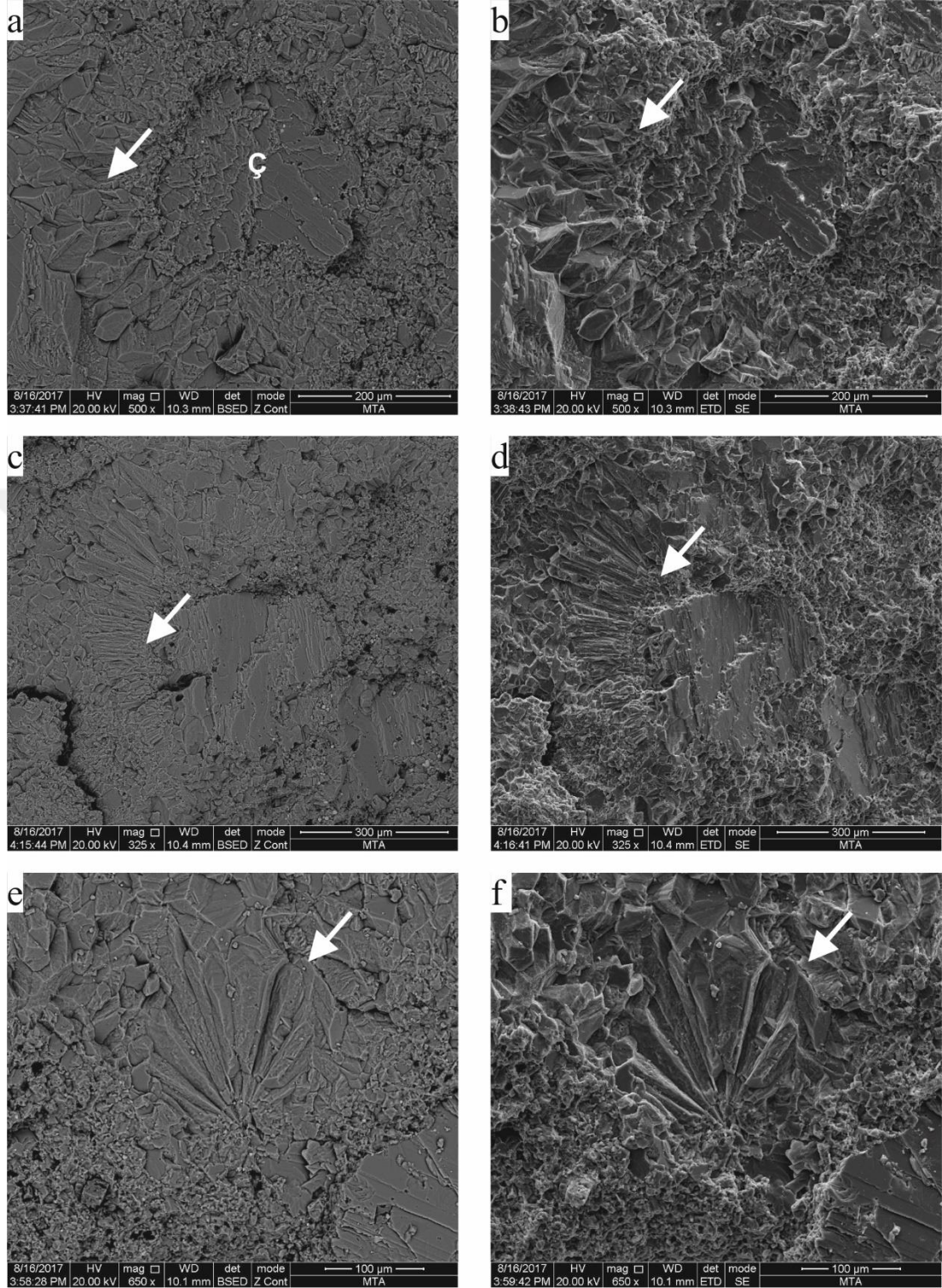
Şekil 4.16. Kemer kesiti oolitic tanetsi-istiftasi fasiyesine (F3) ait SEM görüntüleri; a-b ) ooid çekirdeği (Ç harfi çekirdeği ifade etmektedir) ve çevresinde gözlenen matriksin yeniden kristallenmesi; c-d ) ooid çekirdeği çevresindeki ışınal kalsit kristalleri; e-f ) ooidlerin zar kısmında görünen yelpaze şeklinde dizilmiş kristaller
