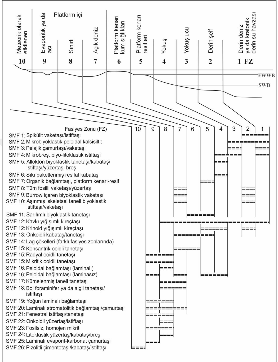
Şekil 3.1. Engelli karbonat platformu üzerindeki Fasiyes Zonlarındaki (Wilson 1975) Standart Mikrofasiyes Tipleri (Flügel 2004). FWWB: Durgun hava dalga tabanı, SWB: Fırtınalı hava dalga tabanı
