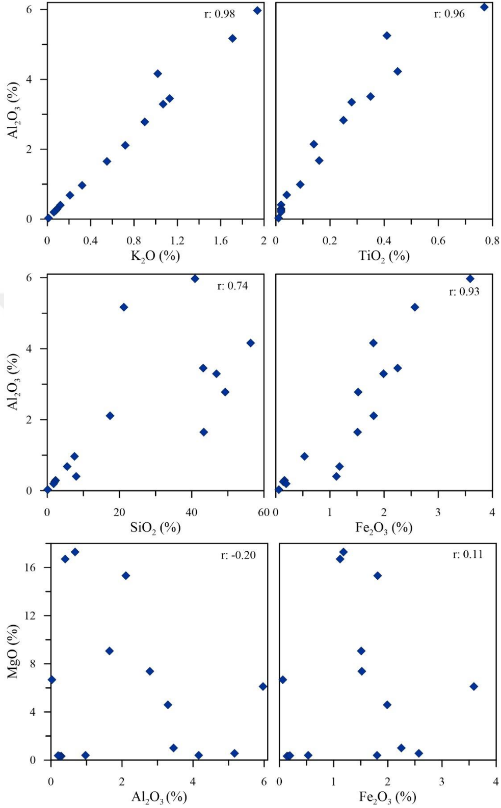
Şekil 4.30. Gazipaşa kesiti örneklerindeki \text{Al}_2\text{O}_3 ile \text{K}_2\text{O} ve \text{TiO}_2 arasındaki ilişki
