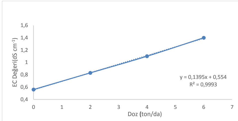
Şekil 4.5. Killi toprağa uygulanan taze atık mantar kompostunun EC değerine etkisi
