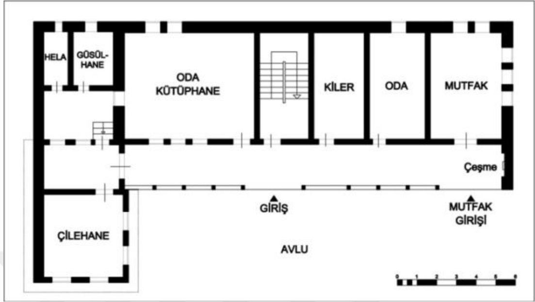
Çizim 4. 3. Emir Sultan Tekkesi Haremi Zemin Kat Planı, Emir Sultan Mh./Bursa, XV. yy., Kübreviyye, Celvetiyye, Nakşibendiyye (Rölevesi)( Taşkın, 63)
