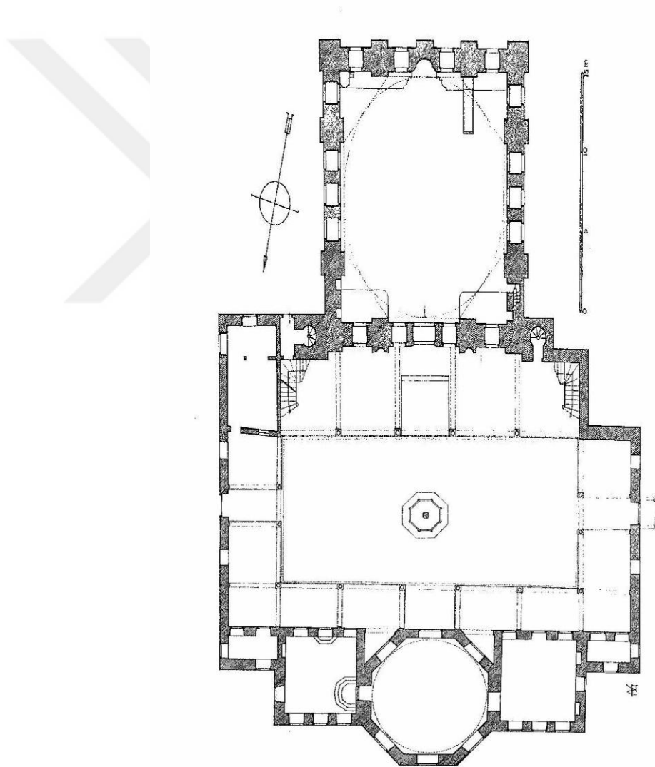
Çizim 4.4. Emir Sultan Cami ve Türbesi (Gabriel) 84
