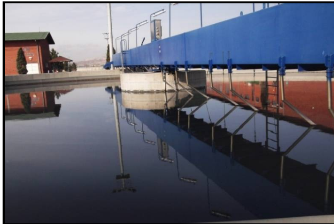
Resim 2.22. Ön çökteltme tankları döner sıyrıcı [58]
