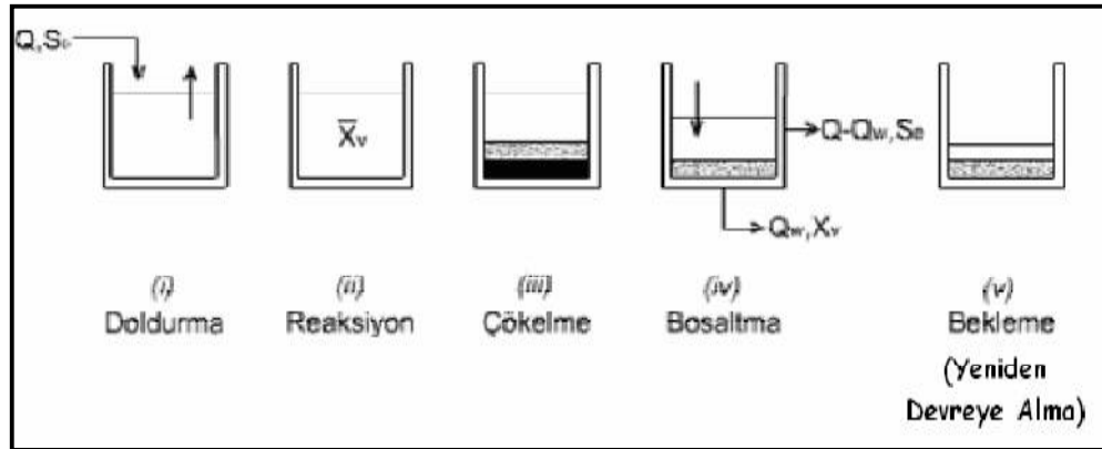
Şekil 2.8. Ardışık kesikli reaktör prosesi çalışma prensibi [53].
