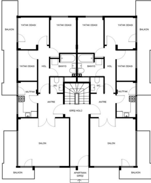
Şekil 3.8. Apartmanın zemin kat planı (1974 tarihli mimari projesi üzerinden şematize edilmiştir).
