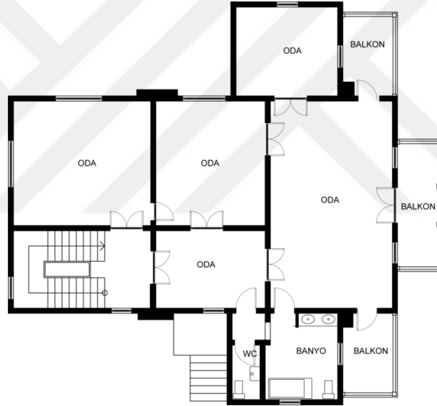
Şekil 3.2. Şaşkın Damat filmindeki ahşap konağın birinci kat planı (2000 yılında çizilen tescil projesinden şematize edilmiştir.)
