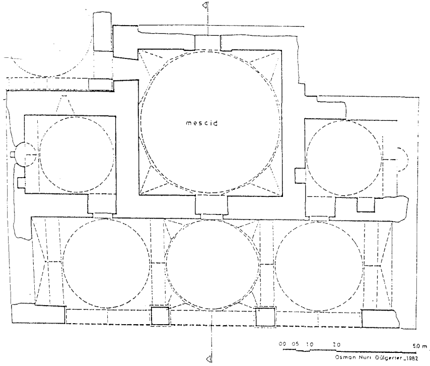
Turhasan Dede Zâviyesi Planı (Dülgerler'den)
