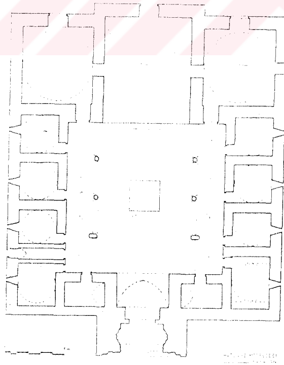
Hâtuniye Medresesi Planı (Sözen'den)
