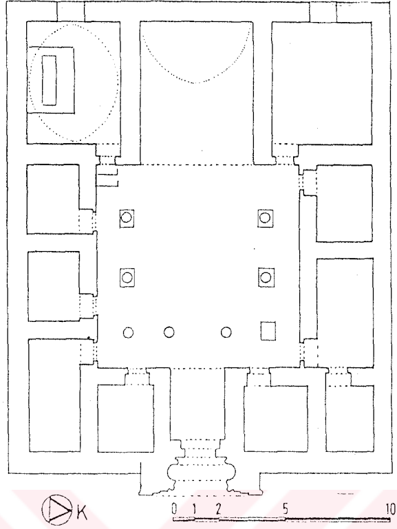
İsmail Ağa (Aka) Medresesi (Taş Medrese) Planı (Dülgerler'den)
