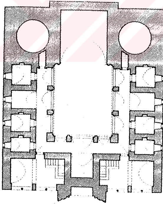
Ak Medrese Alt Kat Planı (Kuran'dan)
