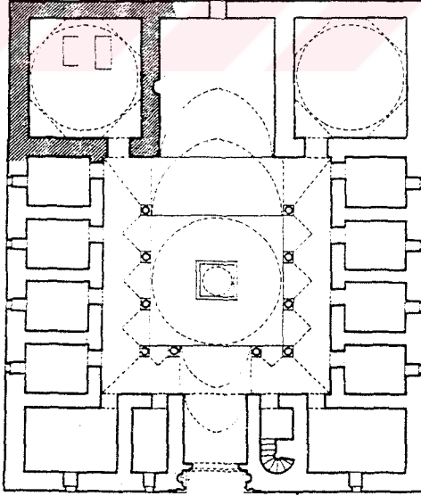
Obaköy Medresesi Planı (Sözen'den)
