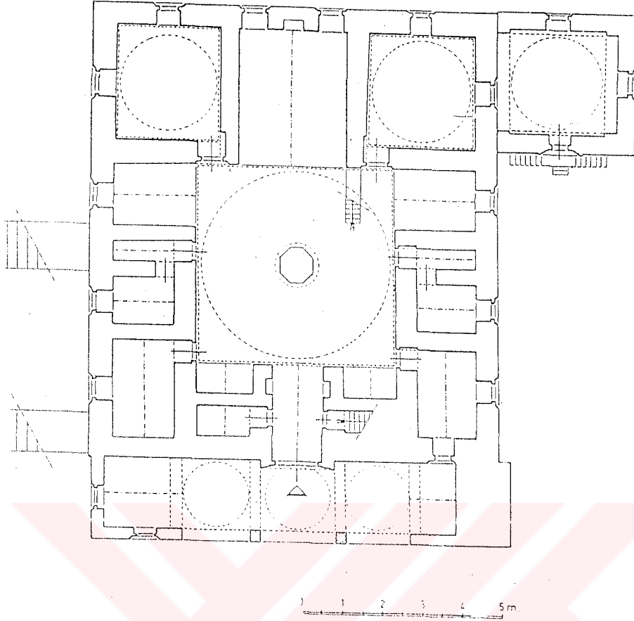
İbrahim Bey İmaret Medresesi Planı (VGMA)
