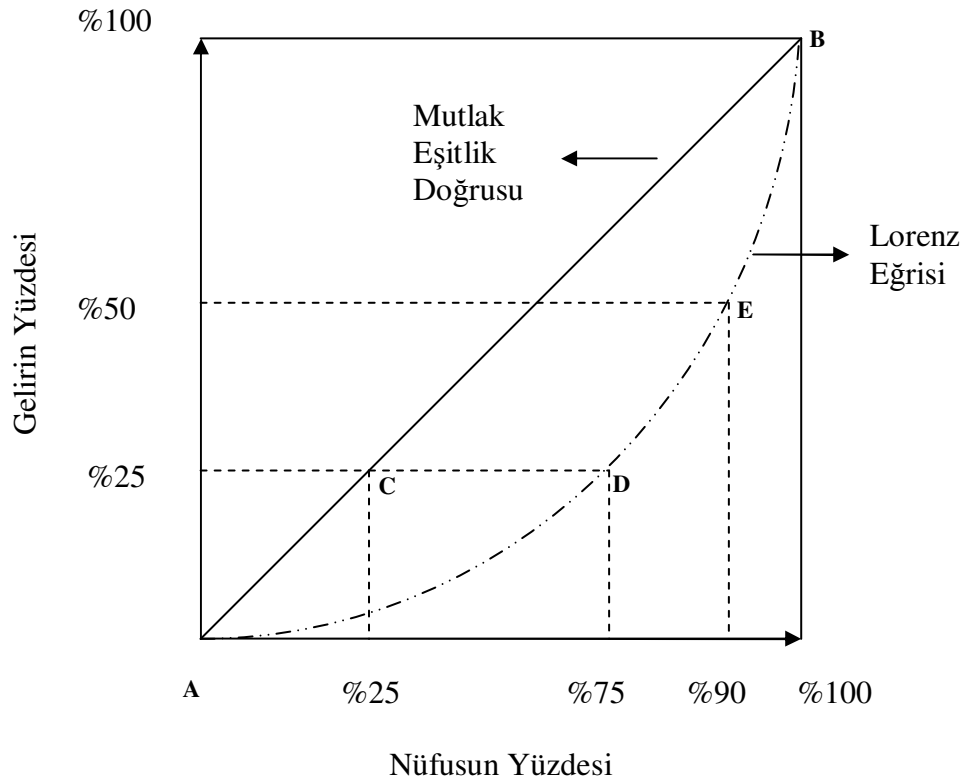
Şekil 1: Lorenz Eğrisi
