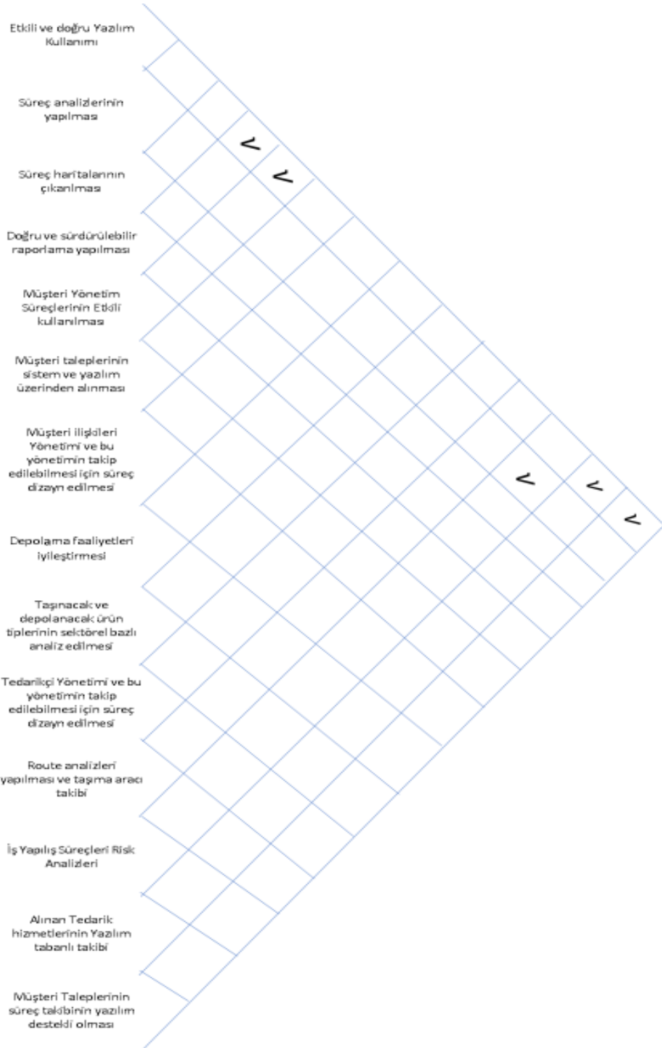
Şekil 4: Çatı Matrisi
