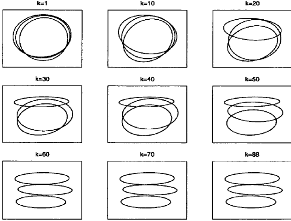
Şekil 3.1. Rasgele başlangıç değerleri kullanılarak EM algoritması için farklı k değerleri için üretilen parametrelere dayalı her alt grup için asimptotik (% 95) elipsoidler grafiği (McLachlan ve Peel, 2000).
