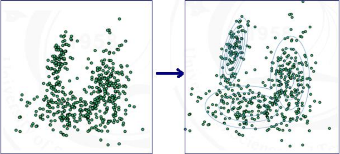
Şekil 3.6. Normal Karışımli model kullanılarak sınıflandırma.
