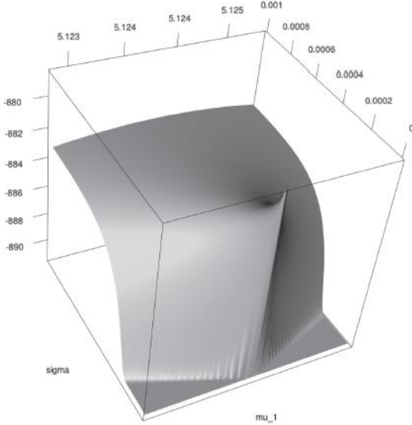
Şekil 3.3. Tek Değişkenli Normal Karışımli Dağılımın Olabilirlik Fonksiyonunun Grafiği (McLachlan ve Peel, 2000).
