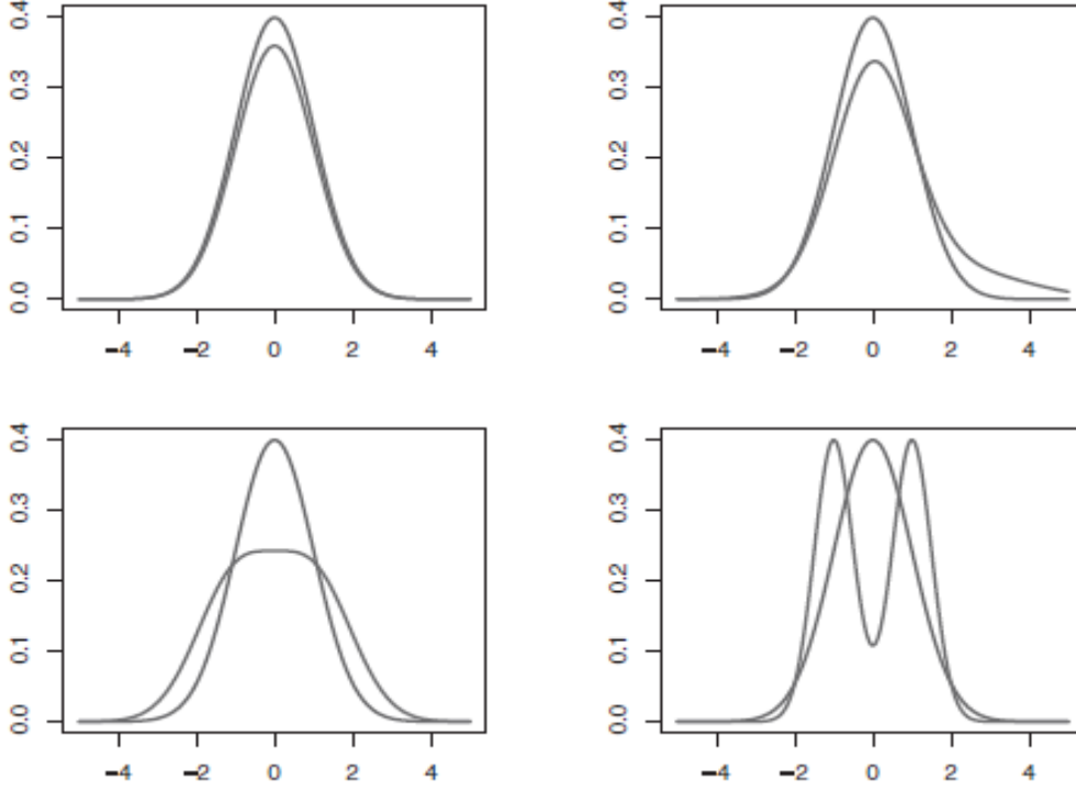
Şekil 3.2. Tek Değişkenli Normal Karışımlılar (McLachlan ve Peel, 2000).
