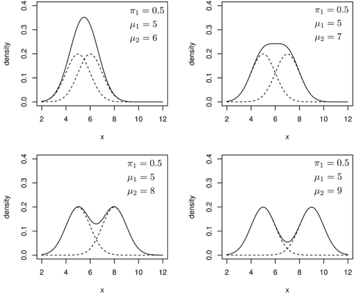
Şekil 3.5. \sigma_1^2 = \sigma_2^2 = 1 ve farklı ortalamalar ( \mu_1, \mu_2 ) için iki değişkenli normal dağılım grafikleri (McLachlan ve Peel, 2000).
