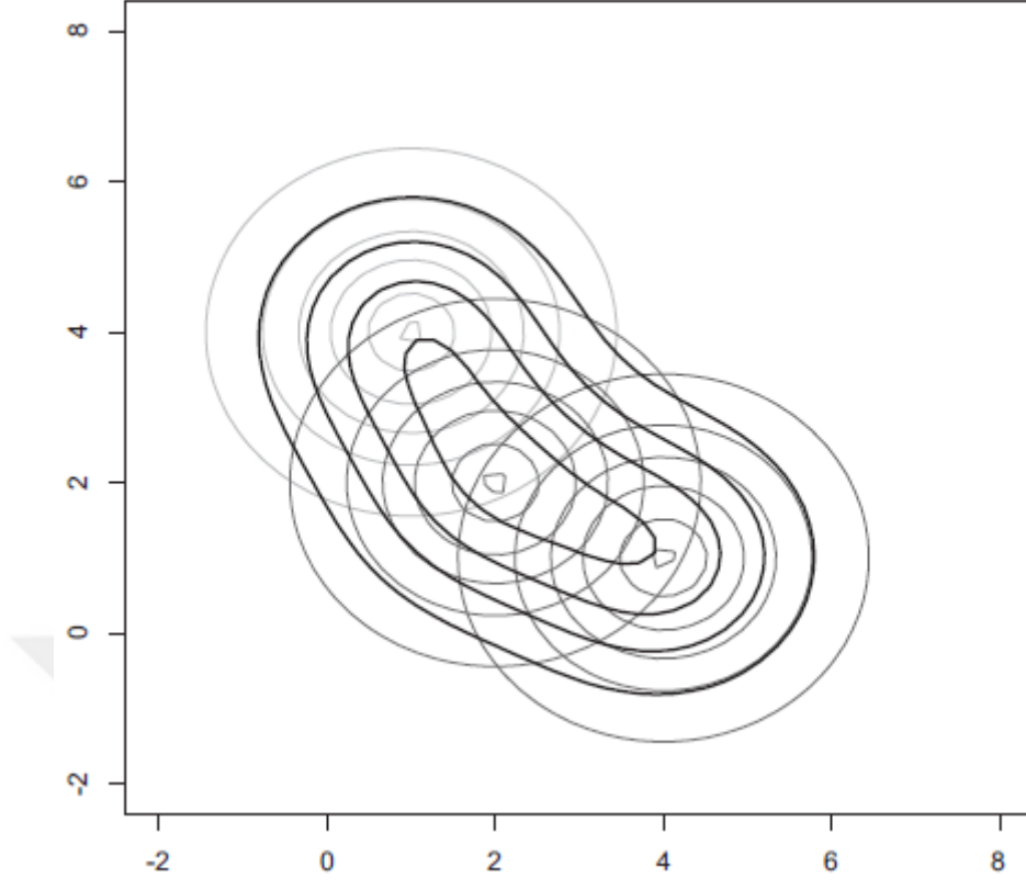
Şekil 3.4. İki Değişkenli Normal Karışımmlılar (McLachlan ve Peel, 2000).
