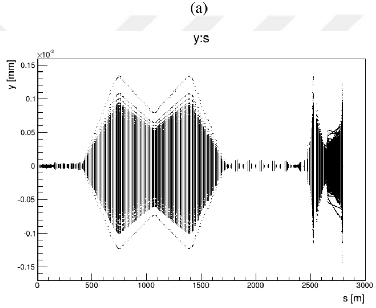
Şekil 4.20. CLIC Demet Taşıma Hattı boyunca demetin yatay (üstte) ve düşey (altta) konumundaki değişim
