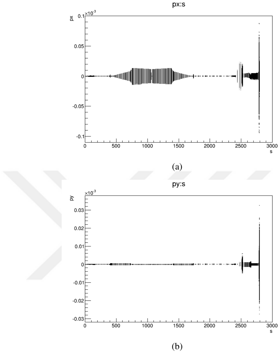
Şekil 4.21. CLIC Demet Taşınım Hattı boyunca demetin yatay (üstte) ve düşey (altta) eksenle yaptığı açıdaki değişim
