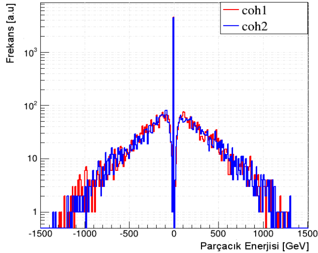
Şekil 4.2. 3000 GeV kütle merkezi enerjisinde oluşan birinci ve ikinci demetin koherent çiftleri
