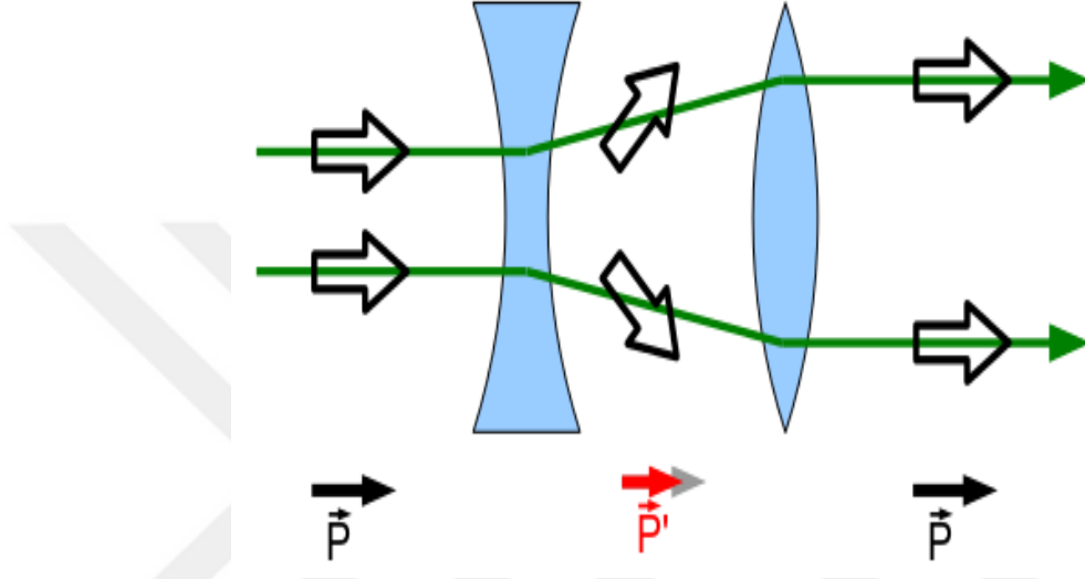
Şekil 2.15. Kuadropol magnet içindeki spin vektörlerinin ( \Rightarrow ) yayılmasının gösterimi
