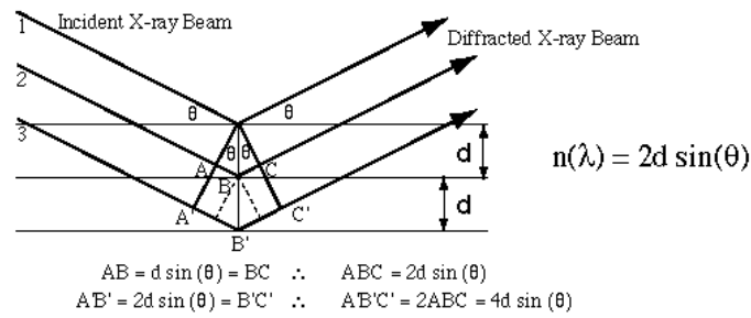
Şekil 3.7. X ışınlarının Kırınımı (Anonim d,2019)
