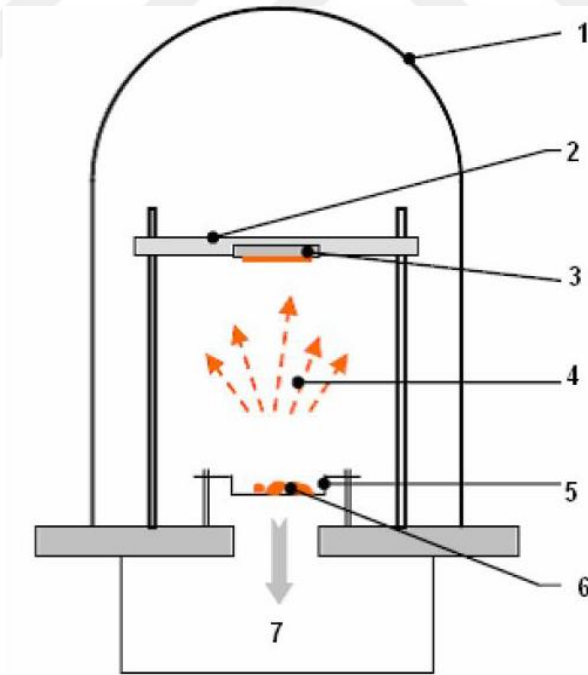
Şekil 3.6. Termal buharlaştırma(rezistans ile) sisteminin şematik gösterilişi 1.Vakum odası 2. Altlık tablası 3. Numune tutucu 4. Metal buharı 5. Isıtıcı filaman 6. Buharlaştırılacak metal (Ocak 2010).
