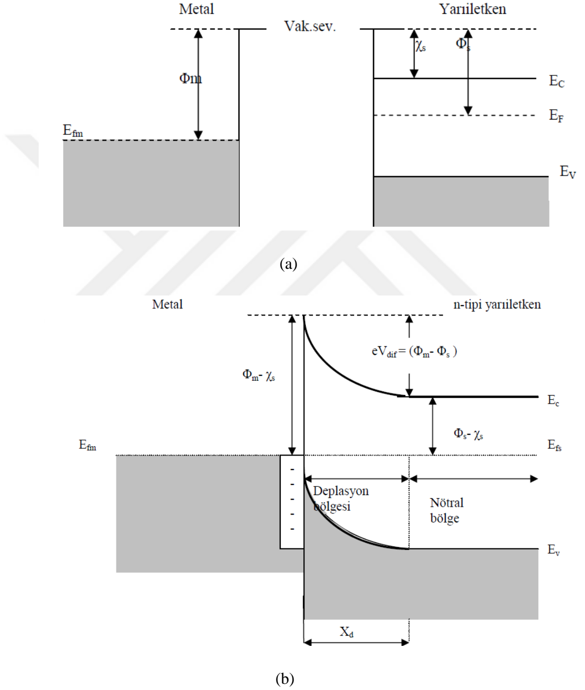
Şekil 2.6. Metal n-tipi yarıiletken omik kontağı a) kontakdan önceki b) kontakdan sonraki enerji band diagramları (Turmuş, 2014)
