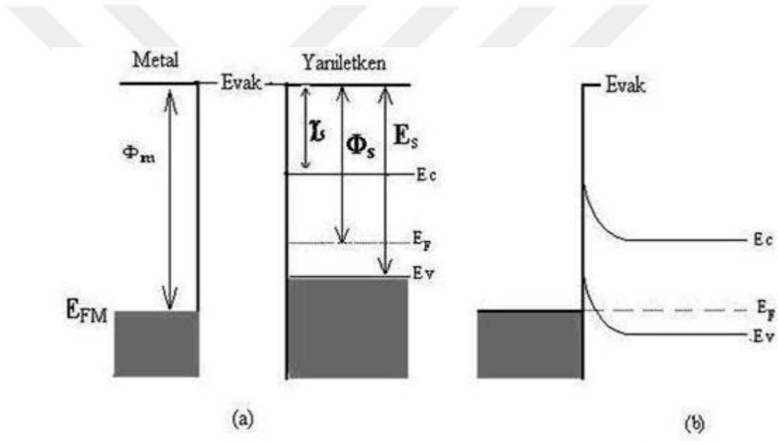
Şekil 2.7. Metal p-tipi yarıiletken omik kontağı:(a) kontakdan önceki,(b) kontakdan sonraki enerji bant diyagramları (Boy, 2013)
