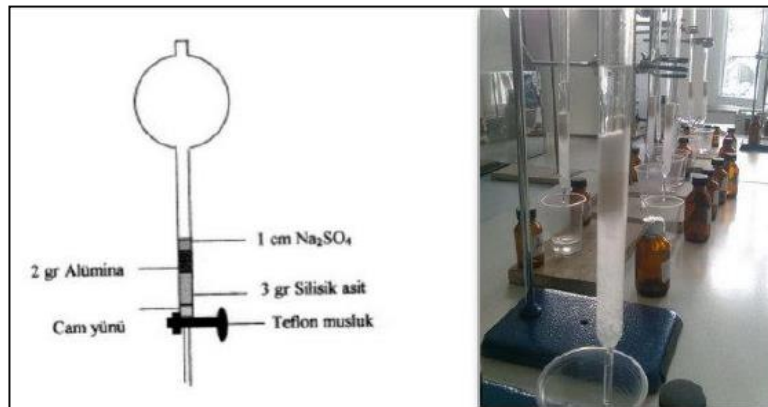
Şekil 3.8. Temizleme kolonu
