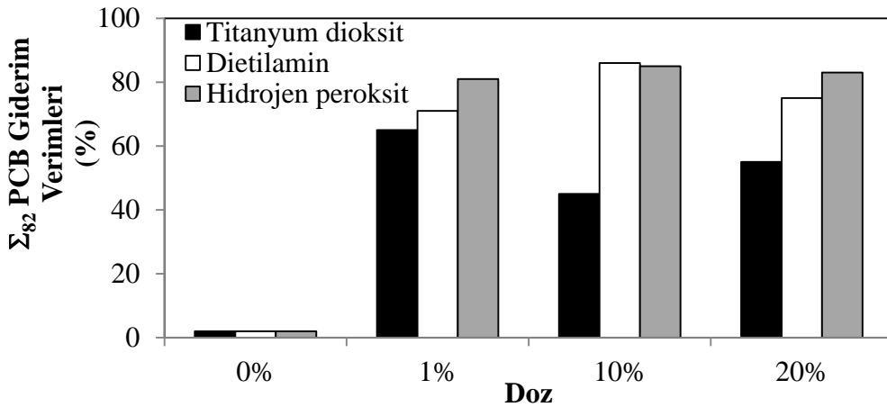
Şekil 4.6. PCB giderim verimlerinin katkı maddesi kullanımıyla değişimi
