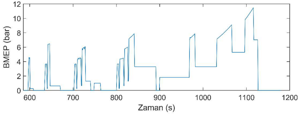
Şekil 4.7. NEDC çevrimi boyunca fren ortalama efektif basıncı (bme p )nın zamana bağlı değişimi
