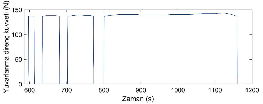
Şekil 4.1. NEDC çevrimi boyunca yuvarlanma direncinin zamana bağlı değişimi
