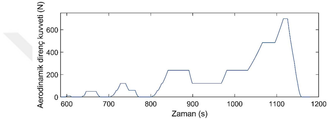
Şekil 4.2. NEDC çevrimi boyunca aerodinamik direnç kuvvetinin zamana bağlı değişimi
