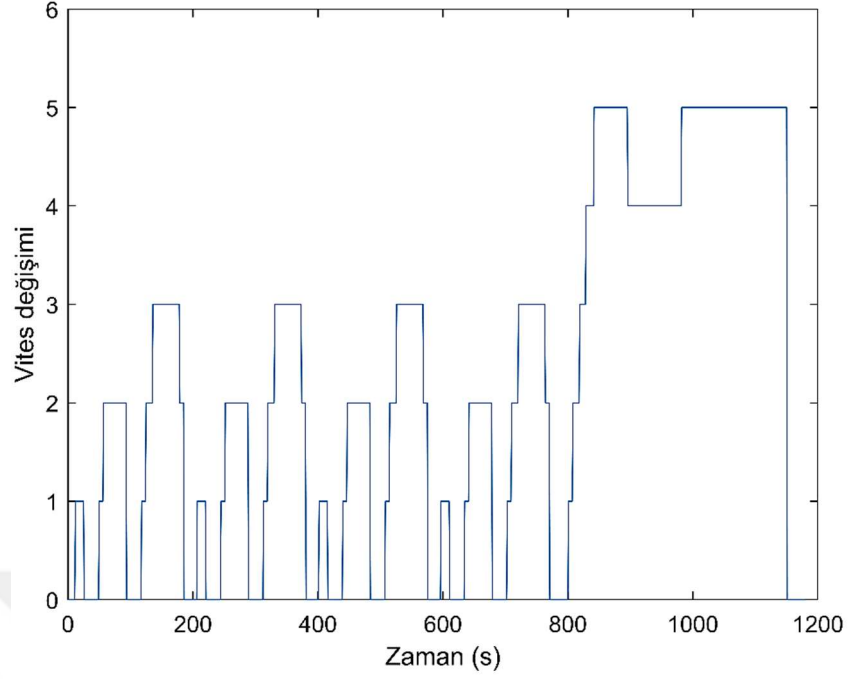
řekil 3.5. NEDC çevrimi boyunca zamana baęlı vites deęiřimi
