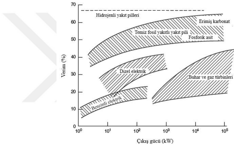
Şekil 2.11. Farklı enerji dönüşüm teknolojilerinin enerji dönüşüm verimi bakımından karşılaştırılması (Li 2007)
