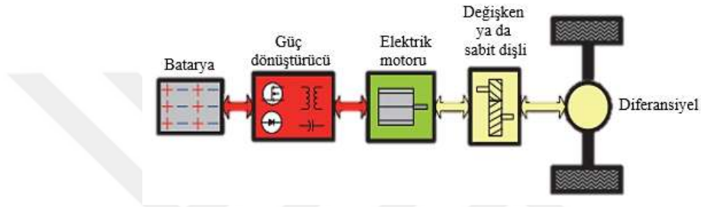
Şekil 2.3. Bataryalı elektrikli aracın yapısı
