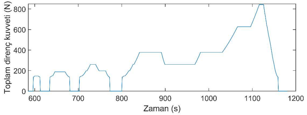
Şekil 4.4. NEDC çevrimi boyunca toplam direnç kuvveti değişimi
