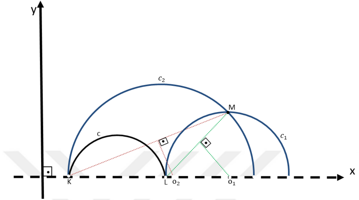
Şekil 3.7. Poincaré üst yarı düzlem modelinde bir yarı çember biçimindeki bir c doğrusuna dışındaki M noktasından çizilen c_1 ve c_2 doğruları
