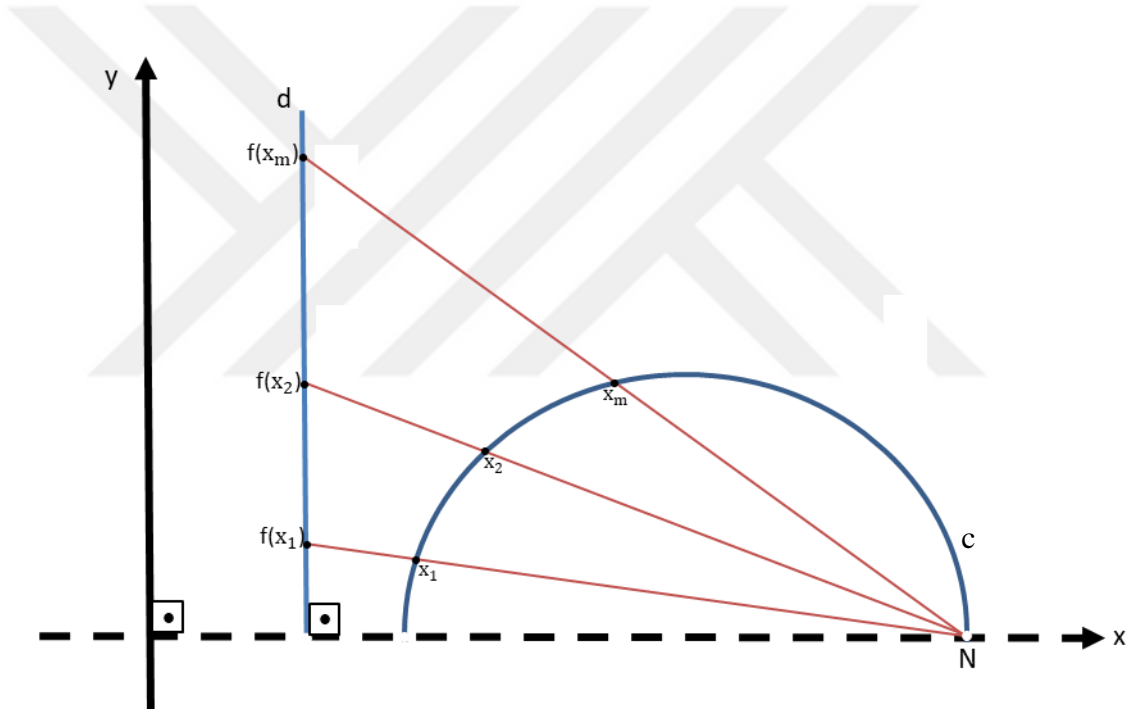
Şekil 3.5. Poincaré üst yarı düzlem modelinin farklı tipteki doğruları üzerindeki noktaların birbirine dönüştürülmesi
