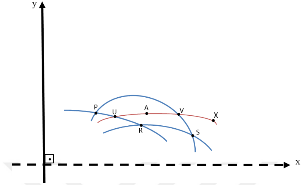
Şekil 3.9. Poincaré üst yarı düzlem modelinin H5 aksiyomu için bir konfigürasyon
