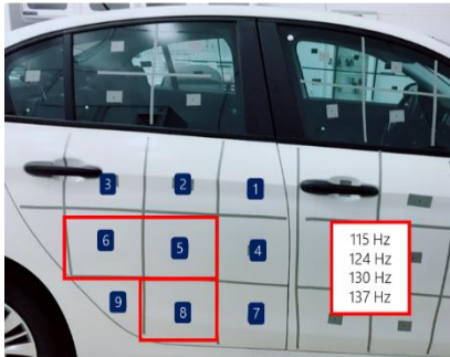
Şekil 4.31. Hesaplanmış arka sağ kapı paneli ve panelciklerin toplam gürültüye olan katkıları
