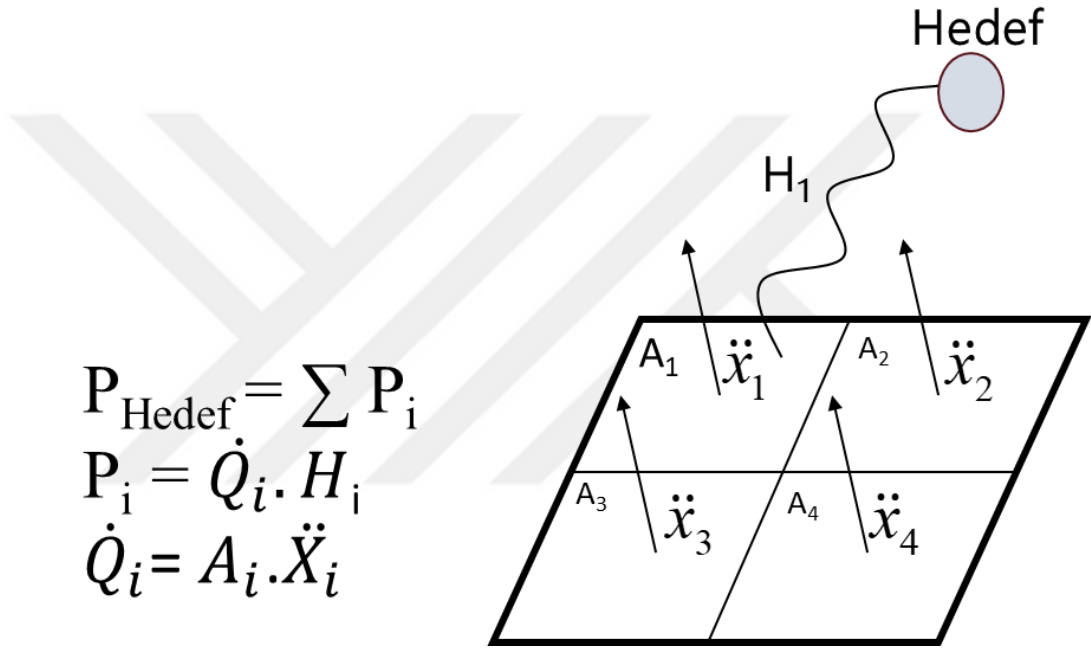
Şekil 3.6. Panel katkı sistematiği
