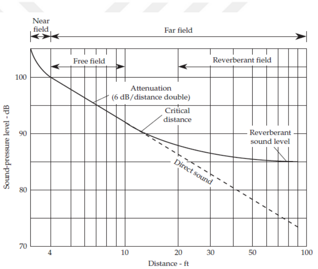
Şekil 2.5. Kapalı hacimlerde ses alanları ve ses basıncı – mesafe ilişkisi (Everest ve Pohlmann 2009)
