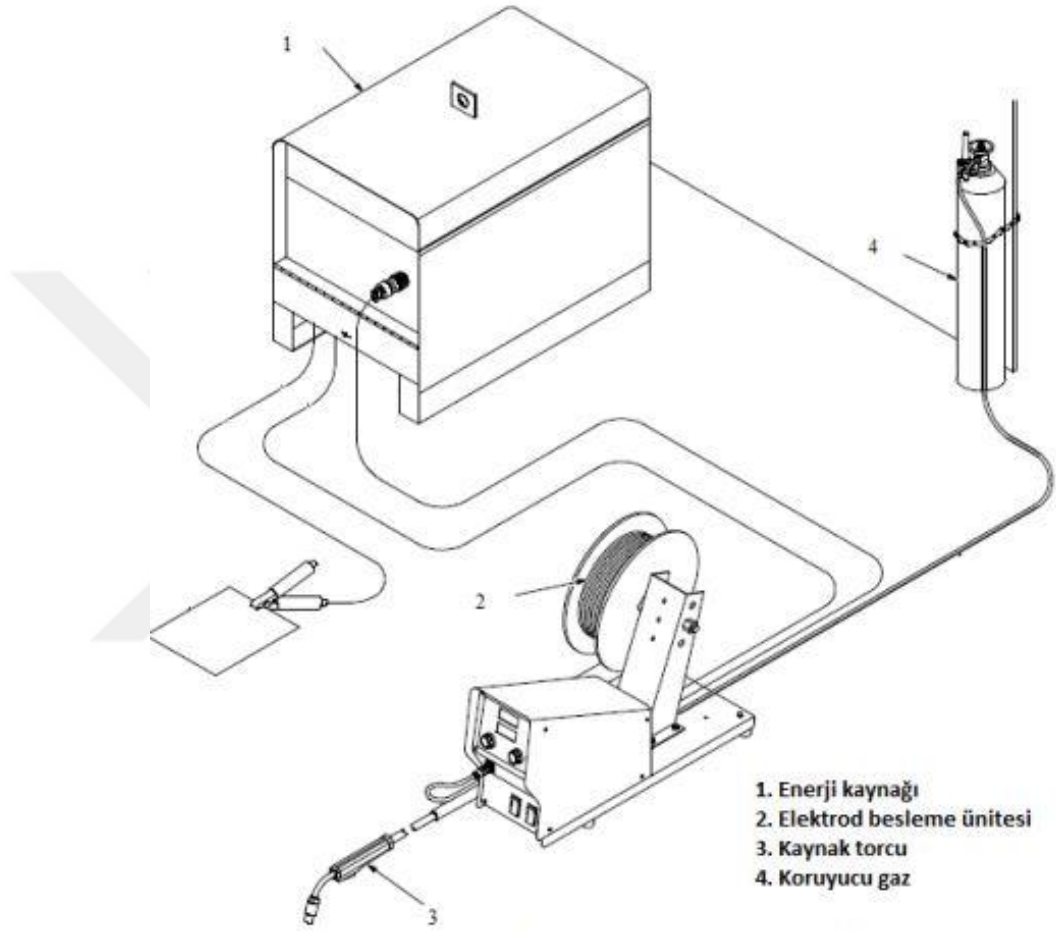
Şekil 2.23. MIG Kaynak ekipmanları (Altuntaş 2015)
