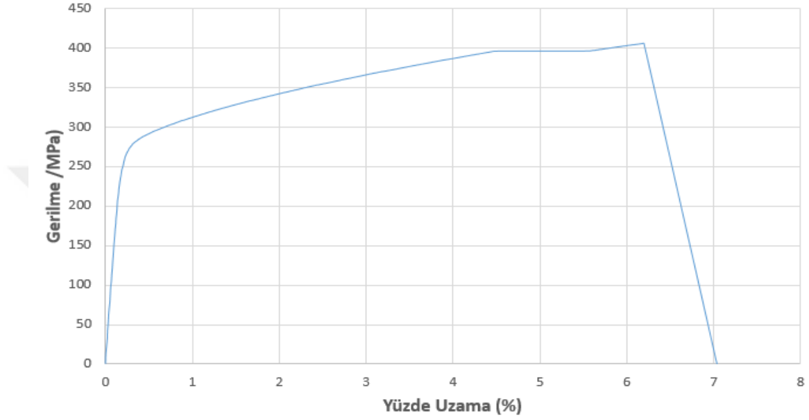
Şekil 4.3. Numune 2 çekme test sonucu
