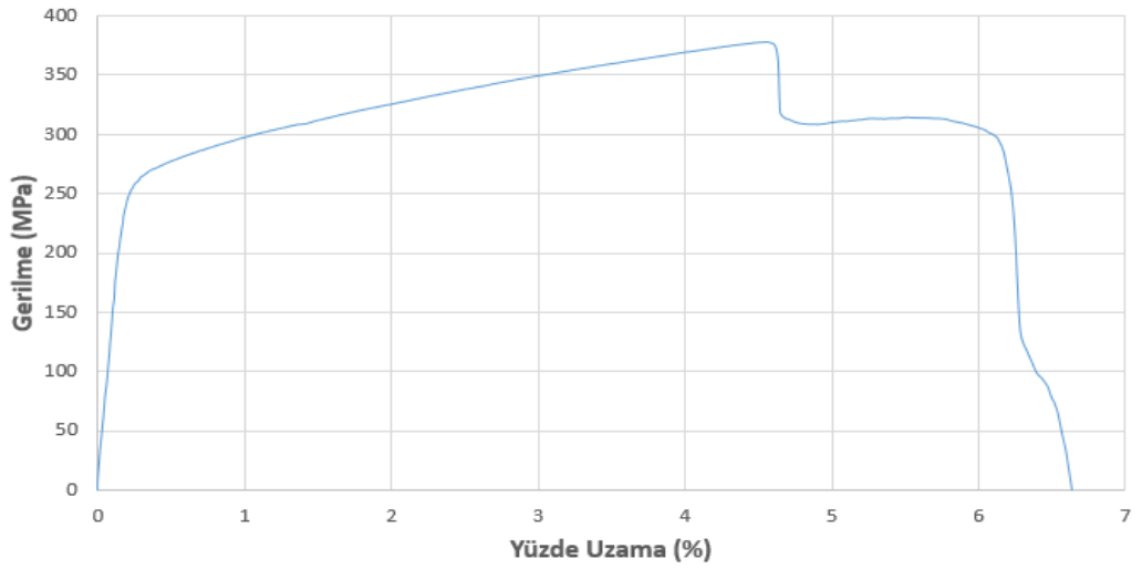
Şekil 4.2. Numune 1 çekme test sonucu
