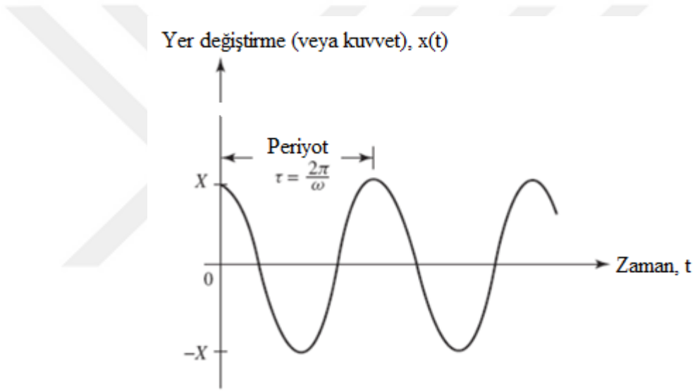
Şekil 3.1. Basit harmonik hareket
