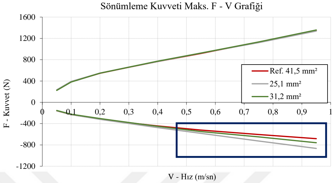
Şekil 4.15. Kapanma çevriminde akış alanları deđiştirilmiş piston kuvvet – hız grafiđi
