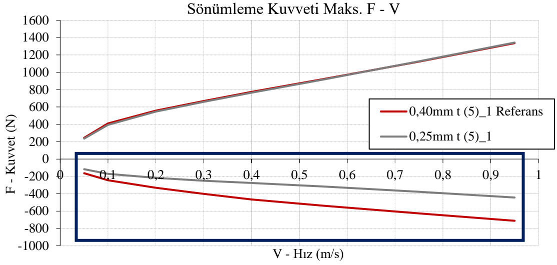
Şekil 4.20. Beş bacaklı parmak yay parçasının kalınlık deęiřimi sonucu meydana gelen sönümlenme kuvveti – hız grafięi
