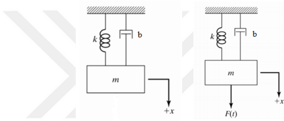
a. Sönümlü serbest titreşim
