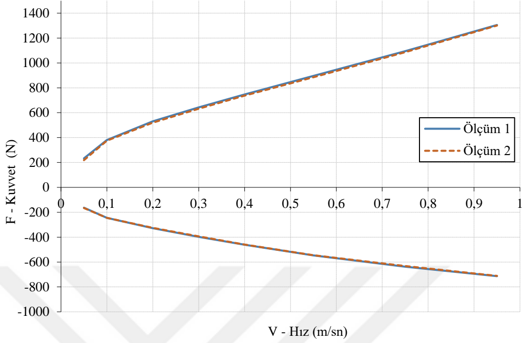
Sönümlenme Kuvveti Maks. F-V Grafiği
