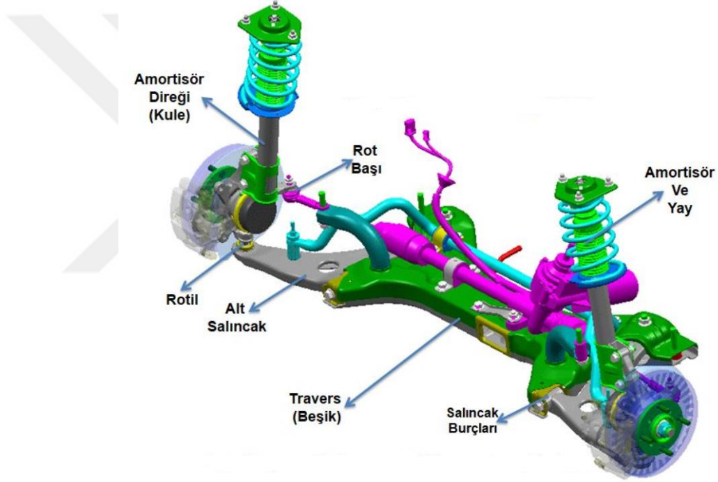
Şekil 3.8. MacPherson bağımsız ön süspansiyon sistemi
