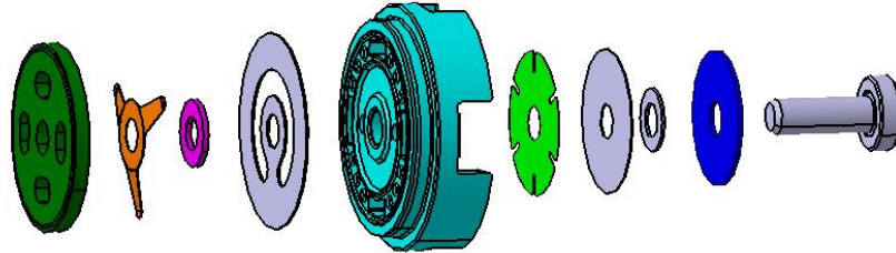
Şekil 3.21. Pullu tip taban valf grubu
