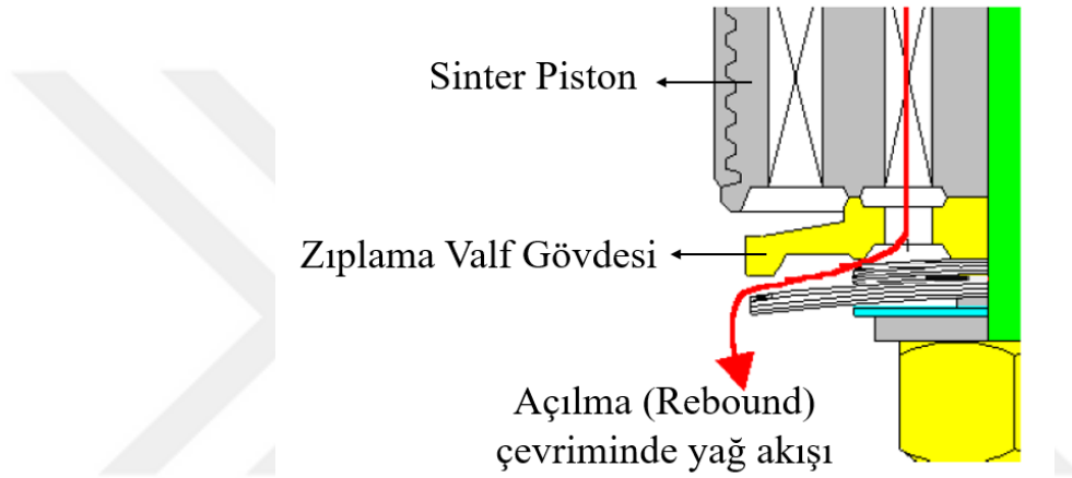
Şekil 4.17. Piston ve zıplama valf gövdesi üzerinde yağ akışı
