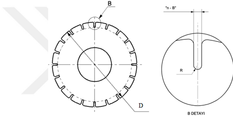
Şekil 4.4. Birinci kademe ayar pulu teknik resim kesit görünüşü
