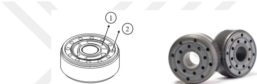
Şekil 3.23. 1: Açılma çevriminde yağ geçişini sağlayan delikler, 2: Kapanma çevriminde yağ geçişini sağlayan delikler
