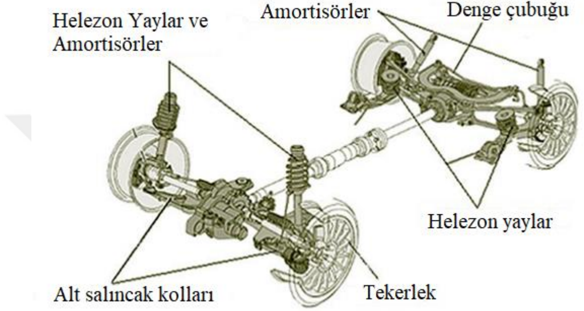
Şekil 2.3. Süspansiyon sistemi elemanları
