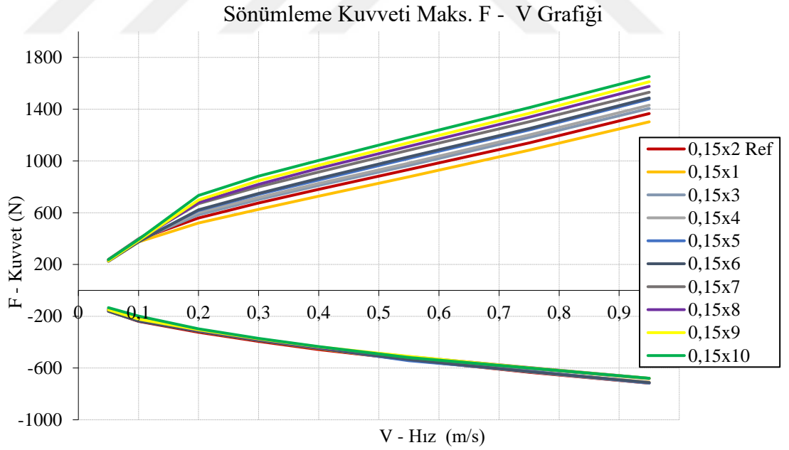
Şekil 4.12. İkinci kademe Ø22 mm pul kalınlığı değiştirilerek elde edilen sönümleme kuvveti – hız eğrileri
