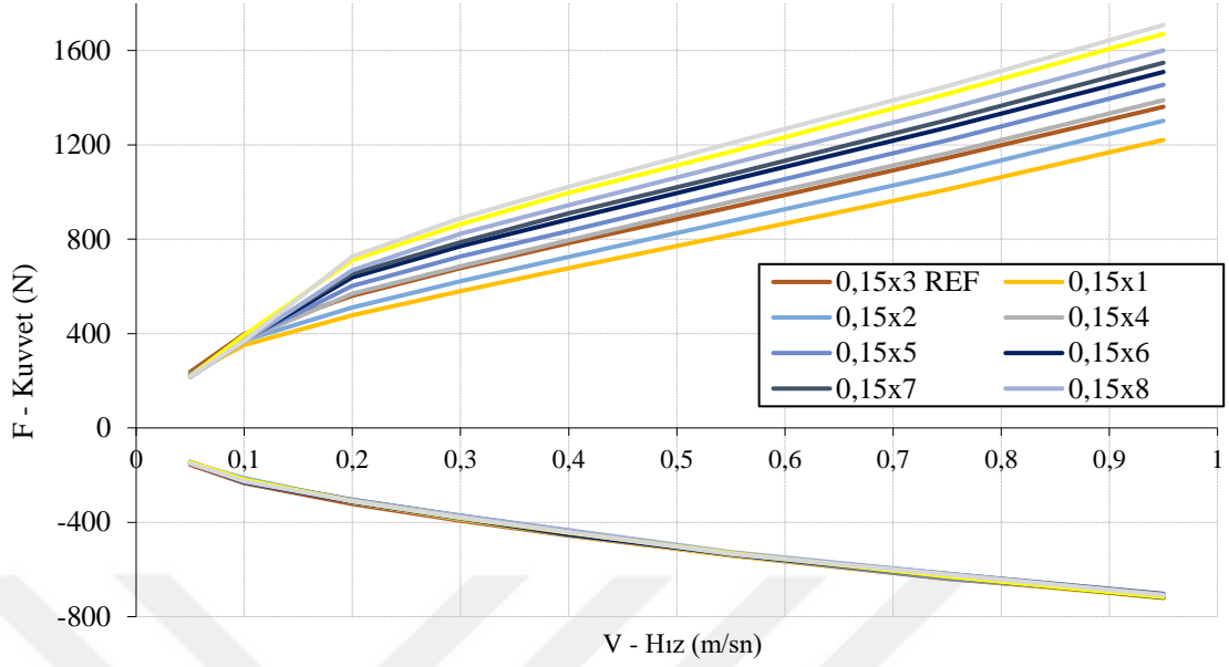
Sönümlenme Kuvveti Maks. F - V Grafiği
