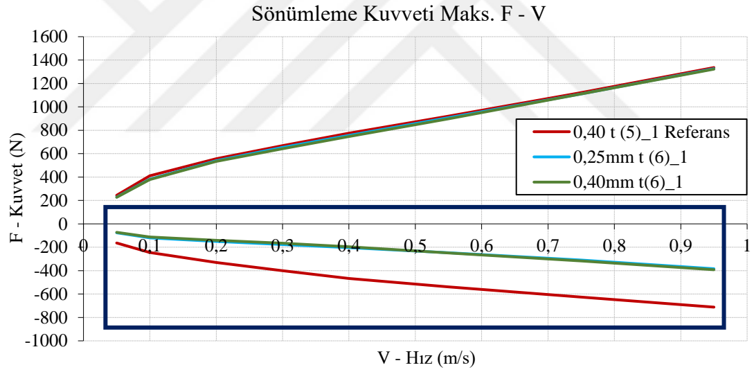
Şekil 4.21. Altı bacaklı parmak yay parçasının kalınlık deęiřimi sonucu meydana gelen sönümlenme kuvveti – hız grafięi
