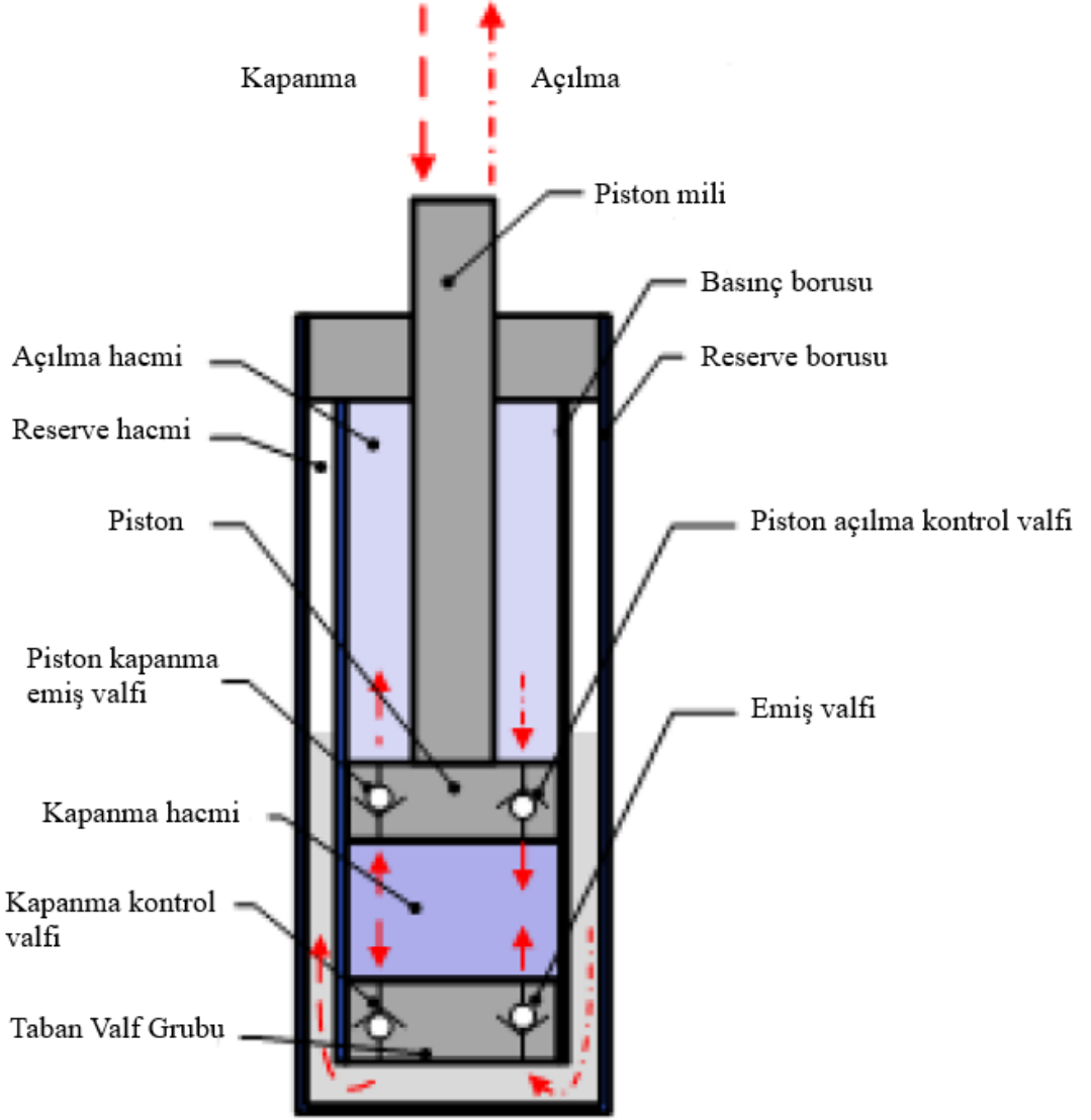
Şekil 2.5. Amortisörün çalışma şekli (Piotr ve ark. 2012'den değiştirilerek alınmıştır.)
