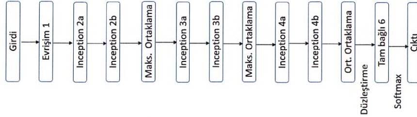
Şekil 3.9 GoogleNet temelli ESA mimarisi
