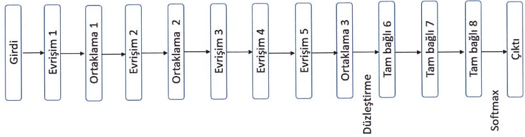
Şekil 3.8 AlexNet temelli ESA mimarisini
