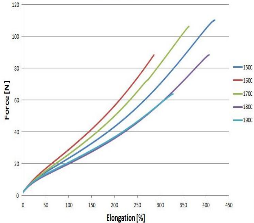
Şekil 4. 17. 10 dk'da B tipi yırtılma numunelerinin farklı sıcaklıklardaki force-elongation test grafikleri
