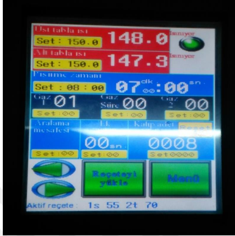
Şekil 3. 12. Vulkanizasyon sıcaklık ve süre panosunun görseli
