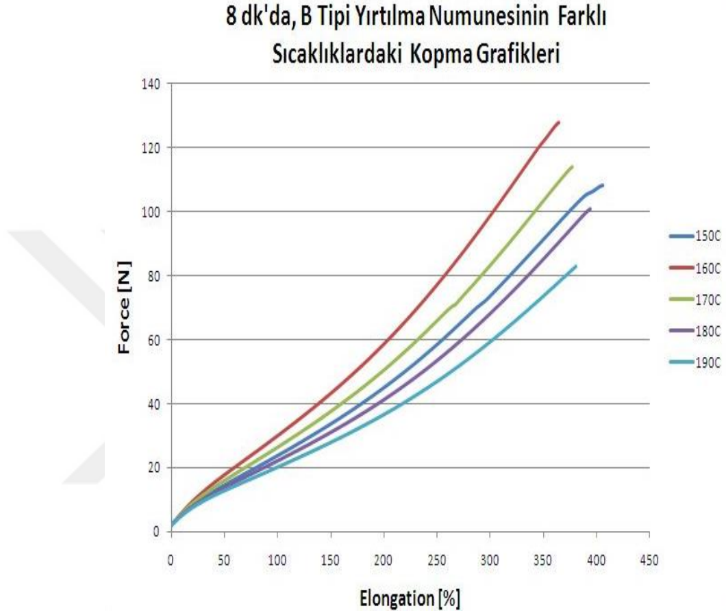
Şekil 4. 16. 8 dk'da B tipi yırtılma numunelerinin farklı sıcaklıklardaki force-elongation test grafikleri
