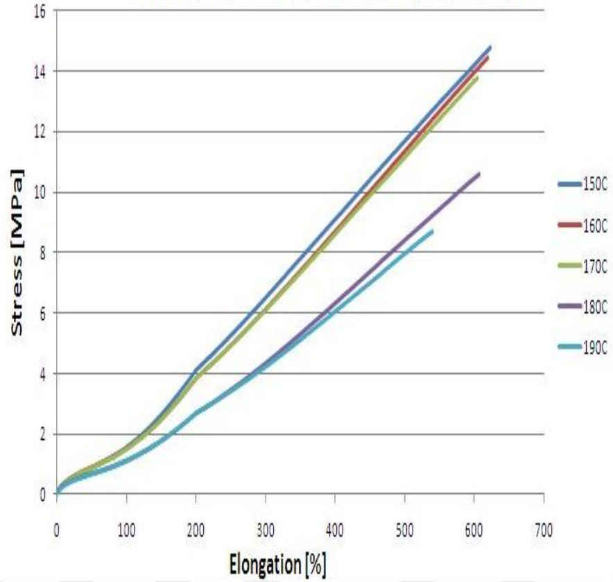
Şekil 4. 8. 12 dk'da farklı sıcaklıklardaki stress-elongation test grafikleri
