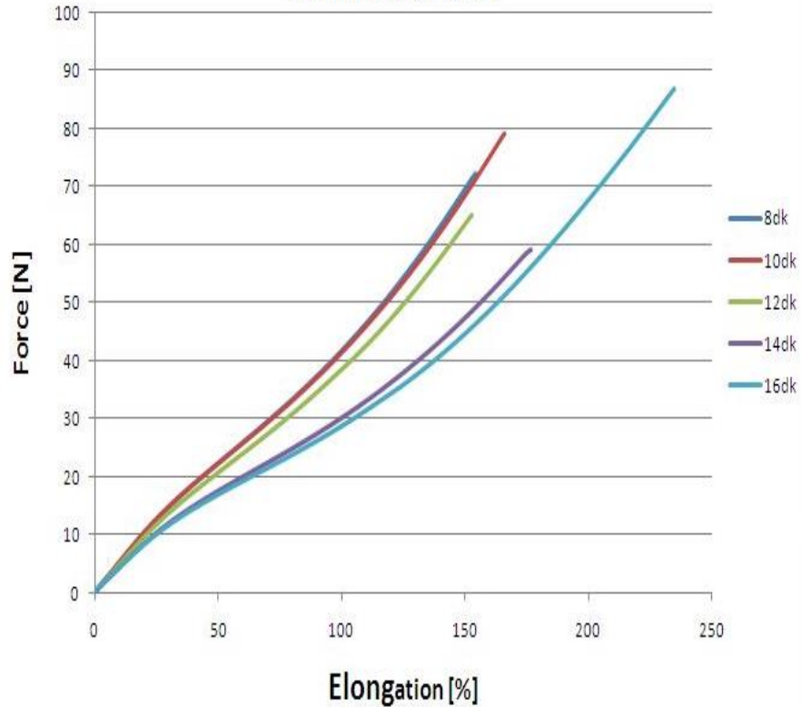
Şekil 4. 23. 170°C'de C tipi yırtılma numunesinin farklı sıcaklıklardaki force-elongation test grafikleri
