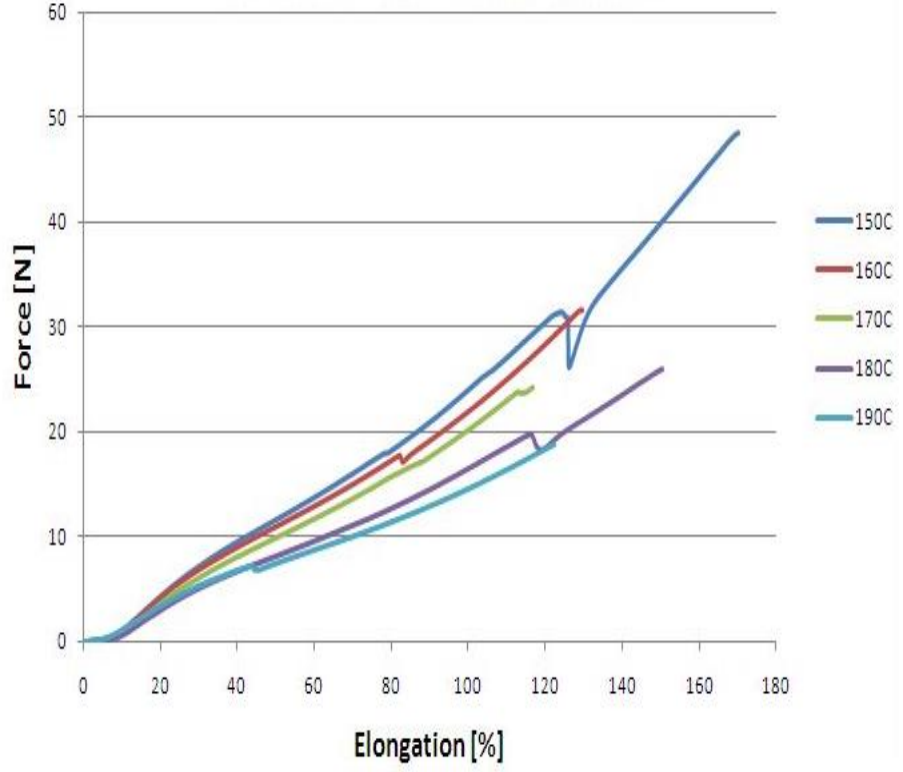
Şekil 4. 38. 12 dk'da T tipi yırtılma numunesinin farklı sıcaklıklardaki force-elongation test grafikleri
