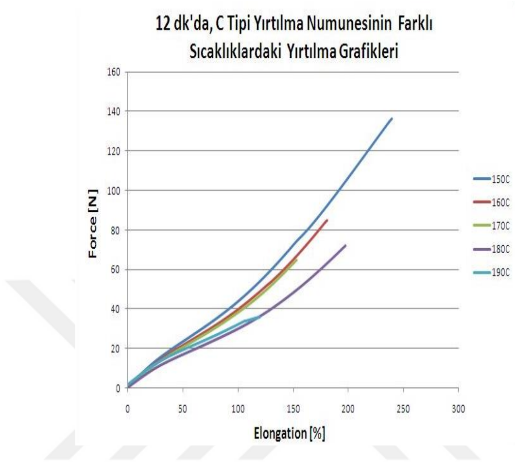
Şekil 4. 28. 12 dk'da C tipi yırılma numunesinin farklı sıcaklıklardaki force-elongation test grafikleri
