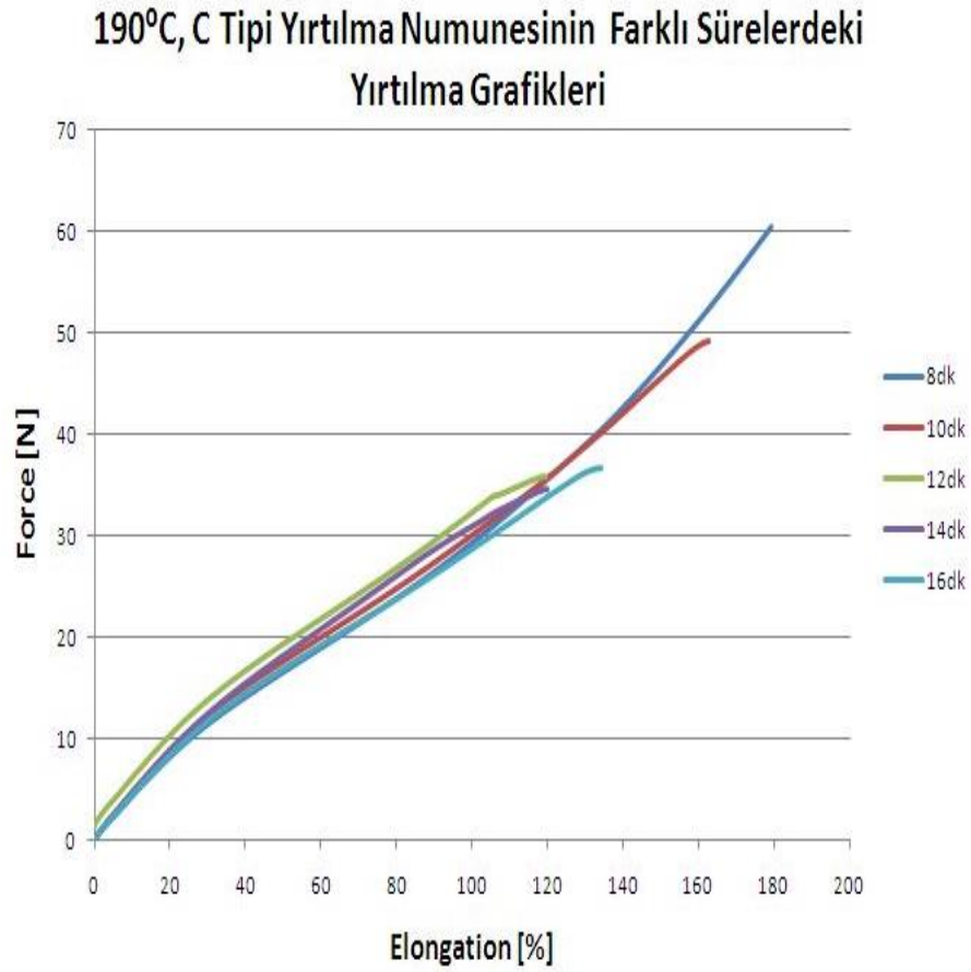
řekil 4. 25. 190°C’de C tipi yırılma numunesinin farklı sıcaklıklardaki force-elongation test grafikleri
