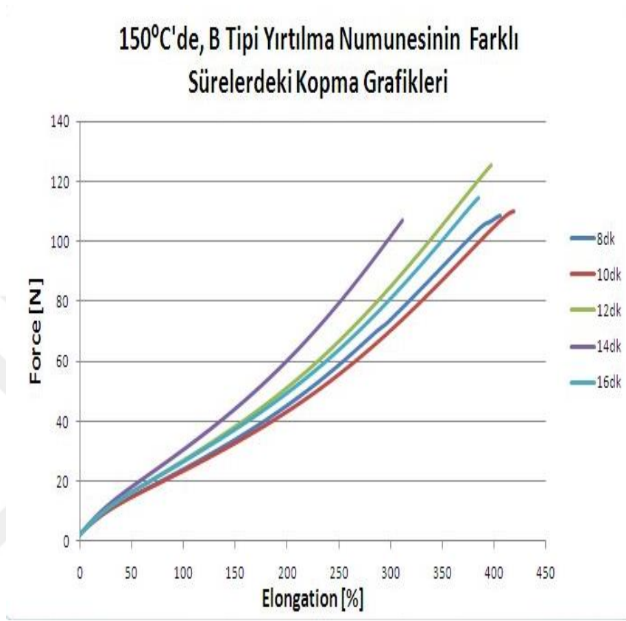
Şekil 4. 11. 150°C'de B tipi yırtılma numunelerinin farklı sürelerdeki force-elongation test grafikleri
