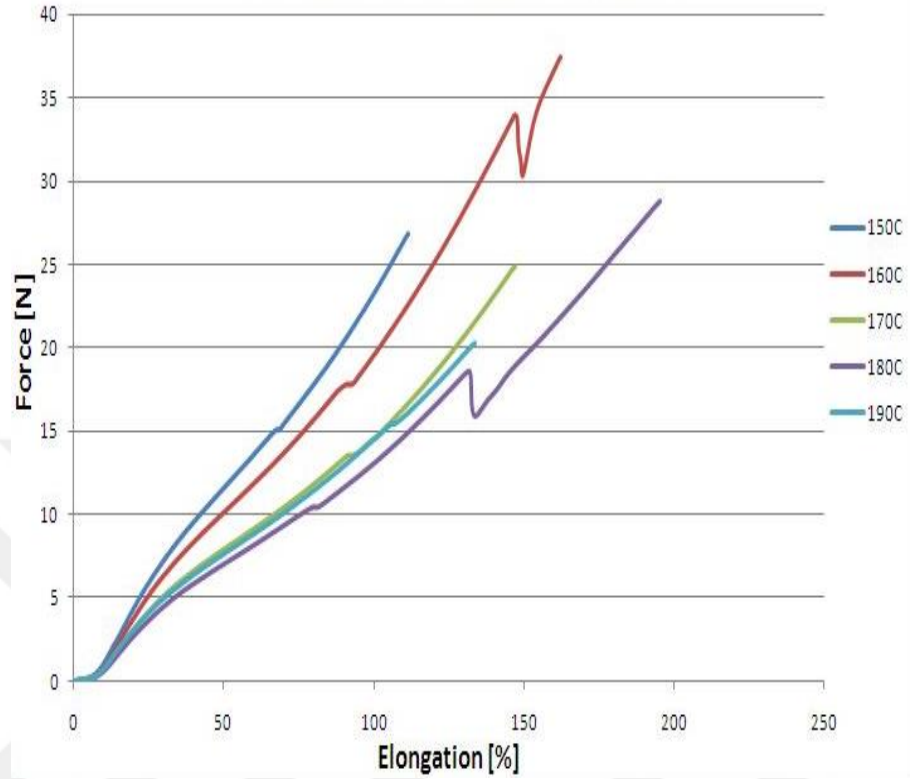
Şekil 4. 40. 16 dk'da T tipi yırılma numunesinin farklı sıcaklıklardaki force-elongation test grafikleri
