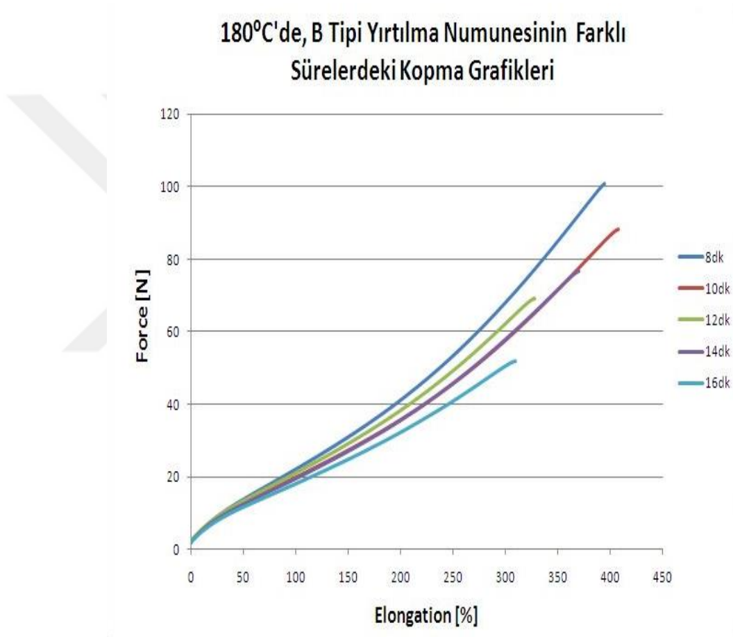
Şekil 4. 14. 180°C'de B tipi yırtılma numunelerinin farklı sürelerdeki force-elongation test grafikleri
