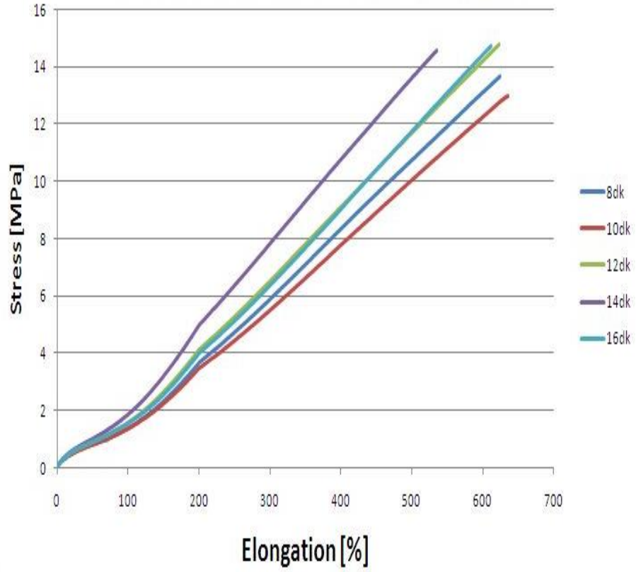
Şekil 4. 1. 150°C’de farklı sürelerdeki gerilme-elongation test grafikleri
