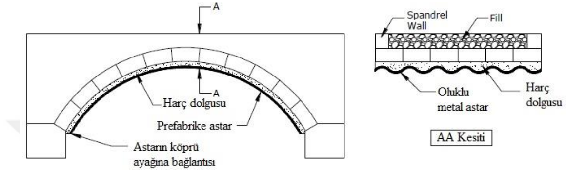
Şekil 3.144. Oluklu metal astar uygulaması (Beuerman 2009)
