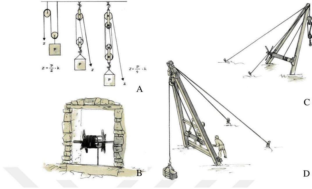
Şekil 3.24. Taşların kaldırılmasında kullanılan çıkırık sistemi 4 a) Makaraların çalışma prensibi b) Basit çıkırık c) Üç kasnaklı sistem d) Kalıcı kablolar ve iki ayaklı sehpa üzerinde basit kaldırma (Barow 2013)
