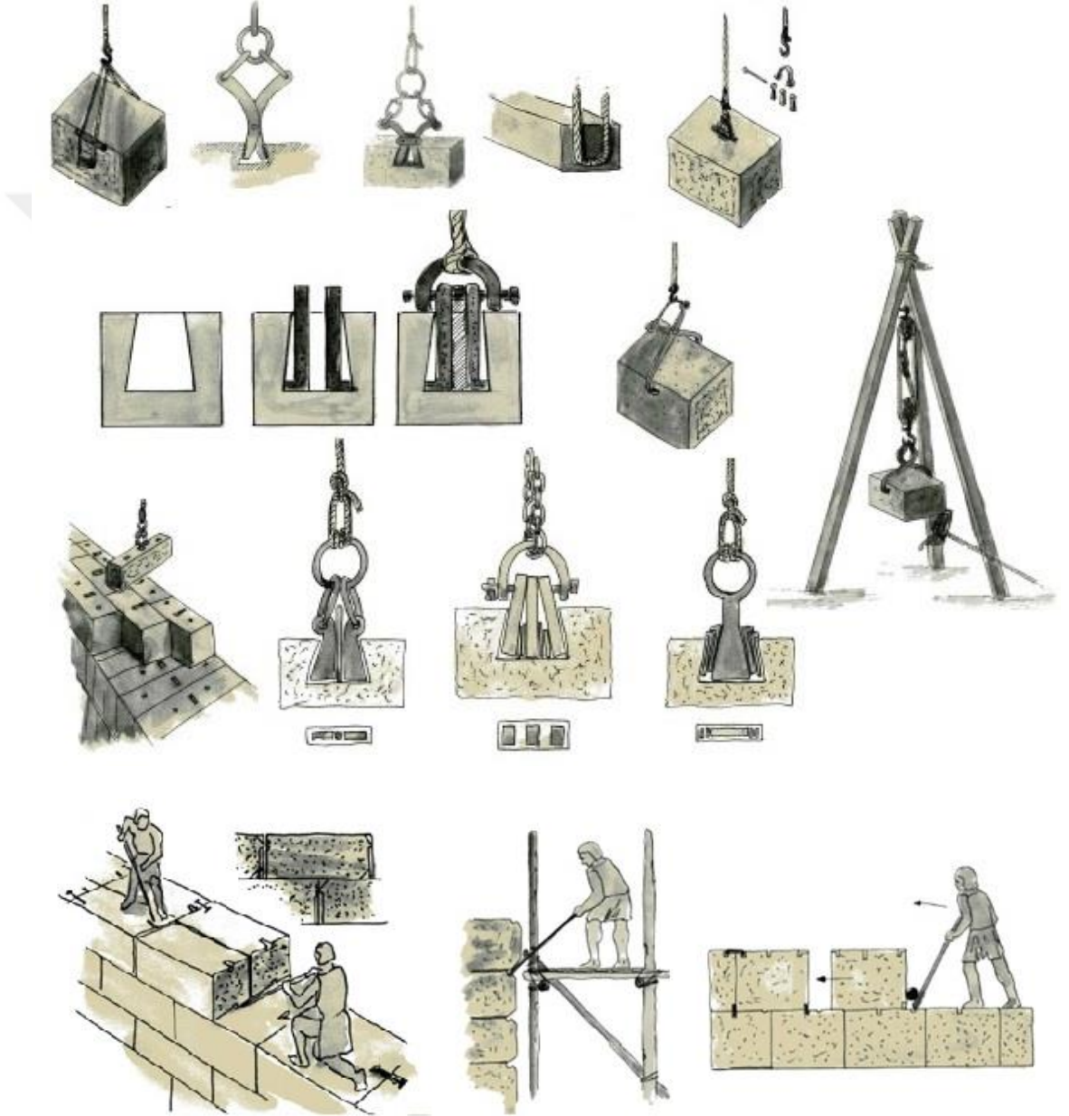
Şekil 3.26. Taşların yerleştirilmesinde kullanılan yöntemler (Barow 2013)
