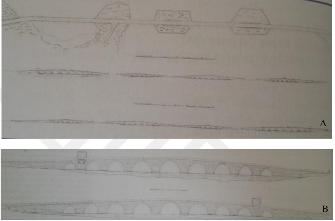
Şekil 3.17. Büyük Çekmece Köprüsü rolövesi a) vaziyet planı ve cephe b) Cephe detayı (Develi 2002)
