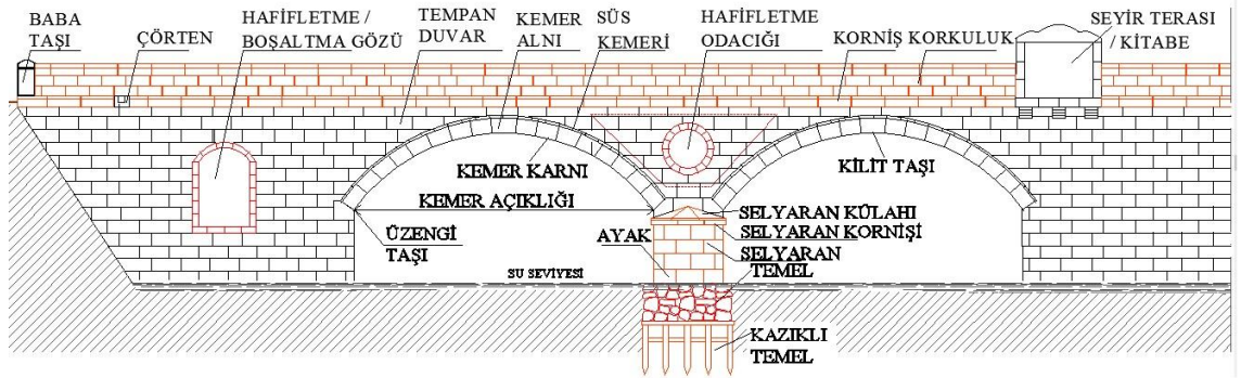
Şekil 3.6. Tarihi köprülere ait terimlerin gösterimi
