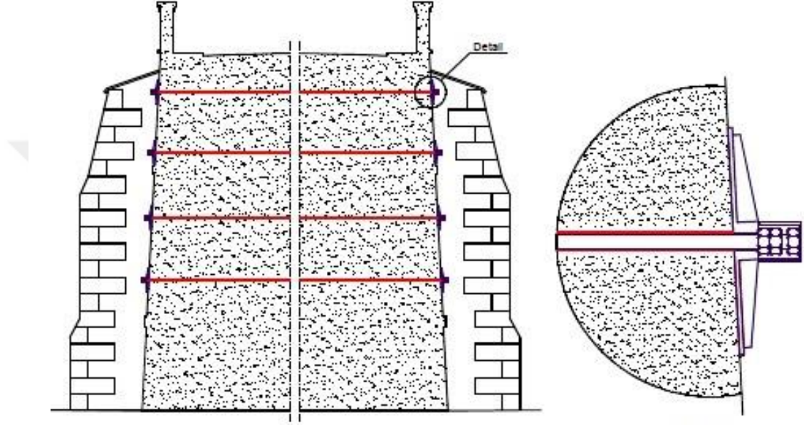
Şekil 3.133. Tarihi Boutaca Köprüsü tempan duvarlarında güçlendirme işleminin görünüş ve detay gösterimi (Oliveira ve Lourenço 2004)
