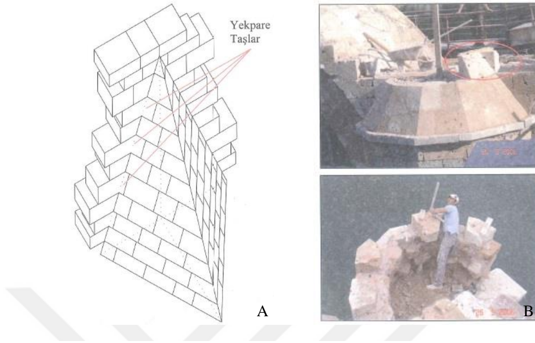
Şekil 3.76. Selyaran yapımı a) Selyaran çizimi b) Konjic Köprüsündeki selyaranın yeniden örülmesi (Sert ve ark. 2009)
