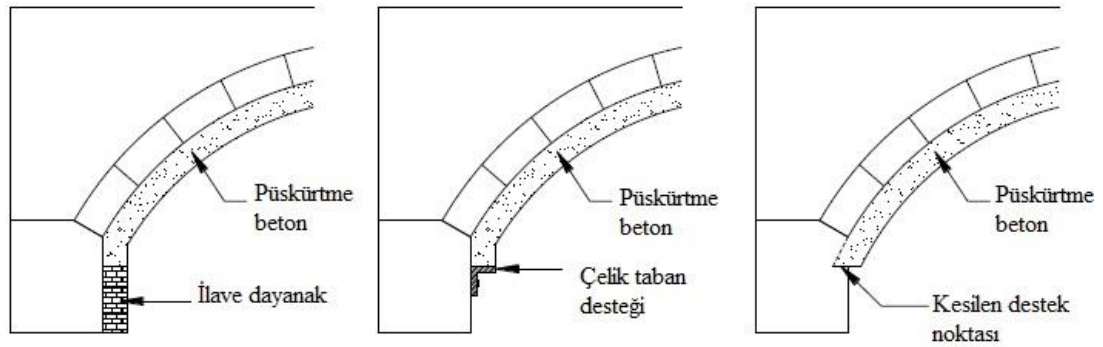
Şekil 3.142. Püskürtme beton uygulama şemaları (Page 1996, Beurman 2009)
