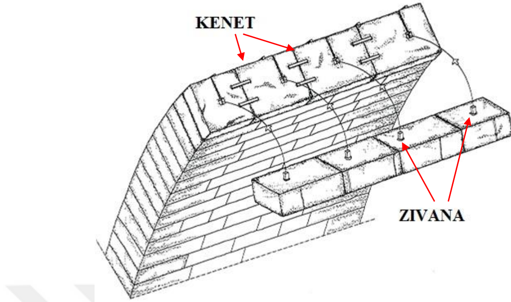
Şekil 3.40. Mostar Köprüsü kemerinde kullanılan kenet ve zivana bağlantıları (Popovac 2006)
