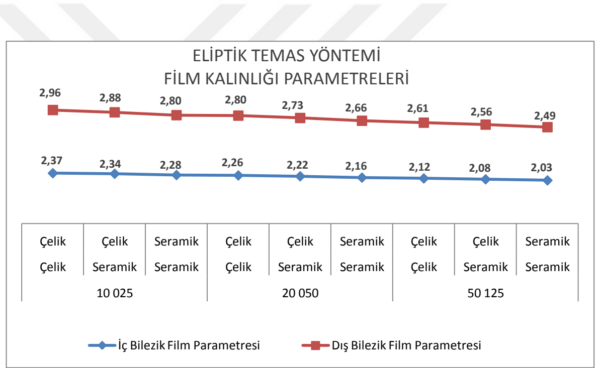
Şekil 5.5. İç ve Dış Bilezik Yüzeylerindeki Film Kalınlığı Parametrelerinin Malzeme Kombinasyonu ve Radyal Yüke Göre Değişimi (Eliptik Temas Yöntemi)
