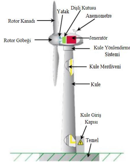
Şekil 2.11. Yatay eksenli türbin yapısı (Koç ve Şenel 2011)
