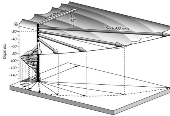
Şekil 2.2. Ekman sipirali (Anonim 2019d)
