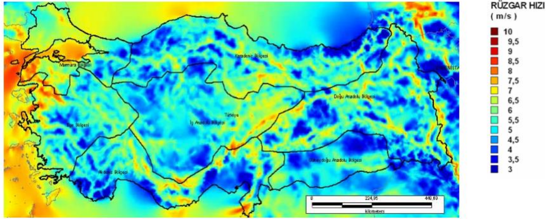
Şekil 3.3. Türkiye geneli 50 metre yükseklikteki ortalama yıllık rüzgâr hızları dağılımı (Anonim 2007)
