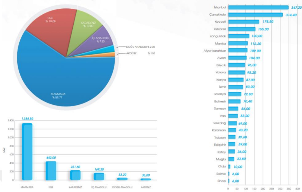
Şekil 2.9. Türkiye lisanslı kurulu güç dağılımları (Anonim 2019g)
