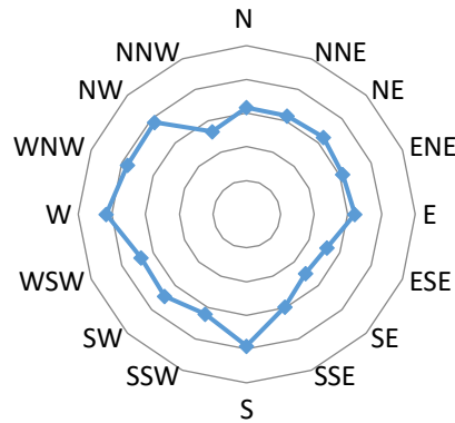
Şekil 4.7. Diyarbakır Çermik ilçe meteoroloji istasyonu rüzgâr esme yönleri
