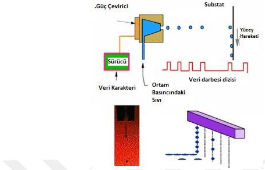
Şekil 2.3. Drop on demand (DOD) ink jet baskı teknolojisi (Anonim 2009)
