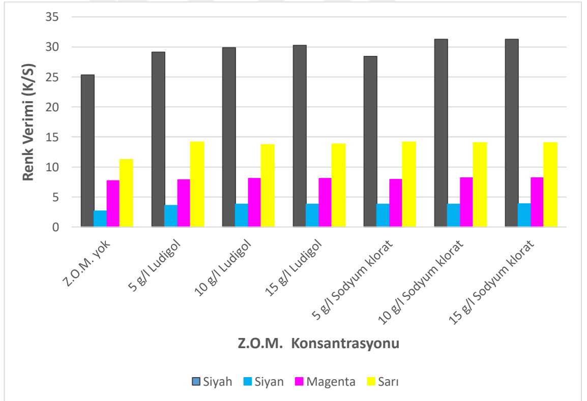
Şekil 4.1. Zayıf oksidasyon malzemesinin renk verimine (K/S) etkisi
