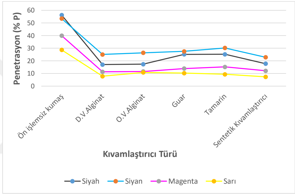
Şekil 4.11. Kıvamlaştırıcı türünün penetrasyon (%P) üzerine etkisi
