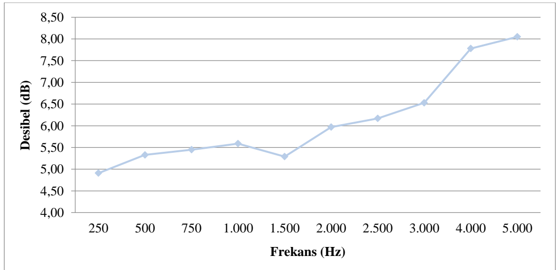
Şekil 4.21. Numune 9 kaplamalı – kaplamalı ters kumaş ses iletim kaybı ölçüm sonucu
