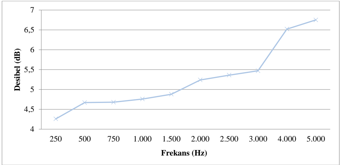
Şekil 4.15. Numune 5 kaplamasız – kaplamasız düz kumaş ses iletim kaybı ölçüm sonucu
