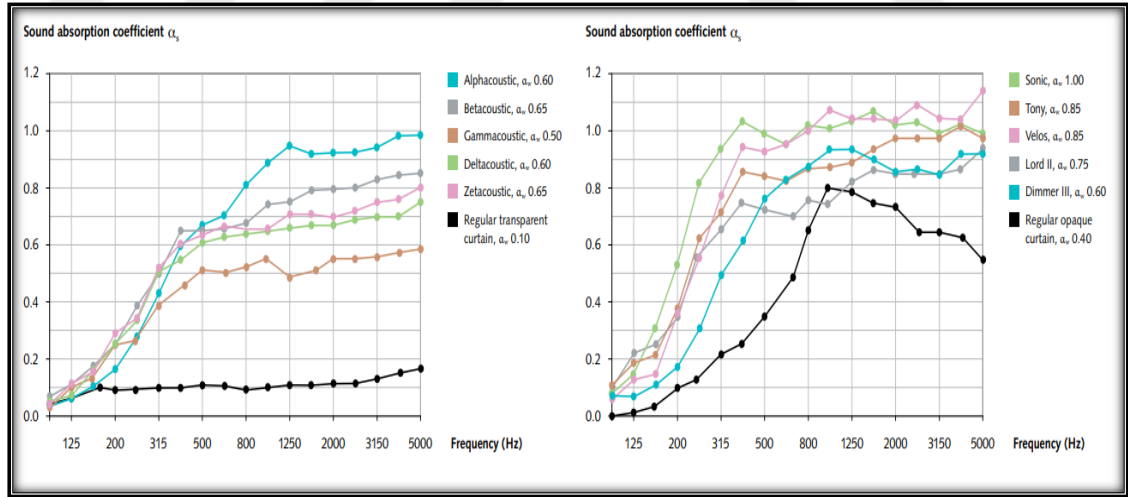
Şekil 2.9. Création Baumann firması tarafından geliştirilen Vario akustik perdenin ses yutumu katsayıları değerleri (Anonim 2019e)
