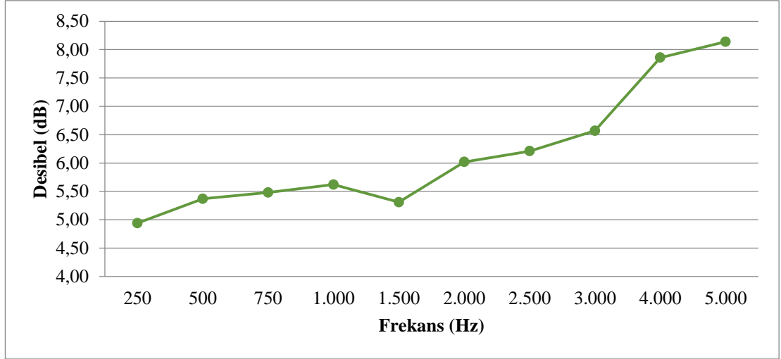
Şekil 4.7. Numune 3 kaplamalı - kaplamalı ters kumaş ses iletim kaybı ölçüm sonucu
