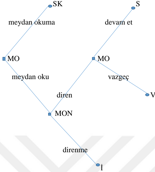
Şekil 4: Ağaç Gösterimi: Devam Et, Vazgeç 313
