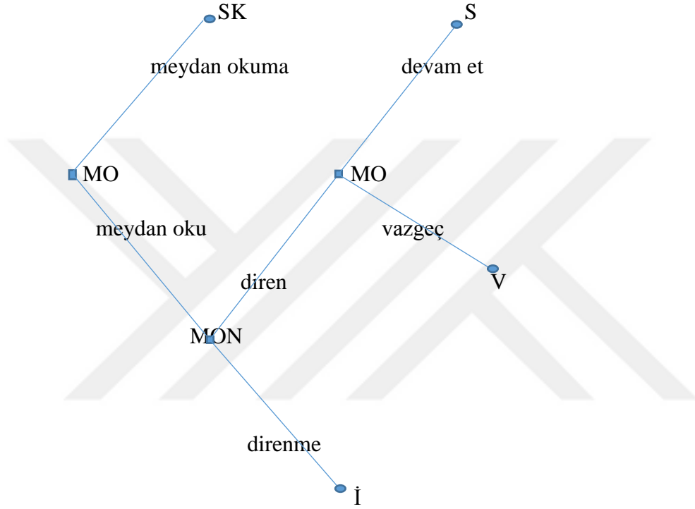
Şekil 7: Çok Stratejili Ağaç Gösterimi 320
