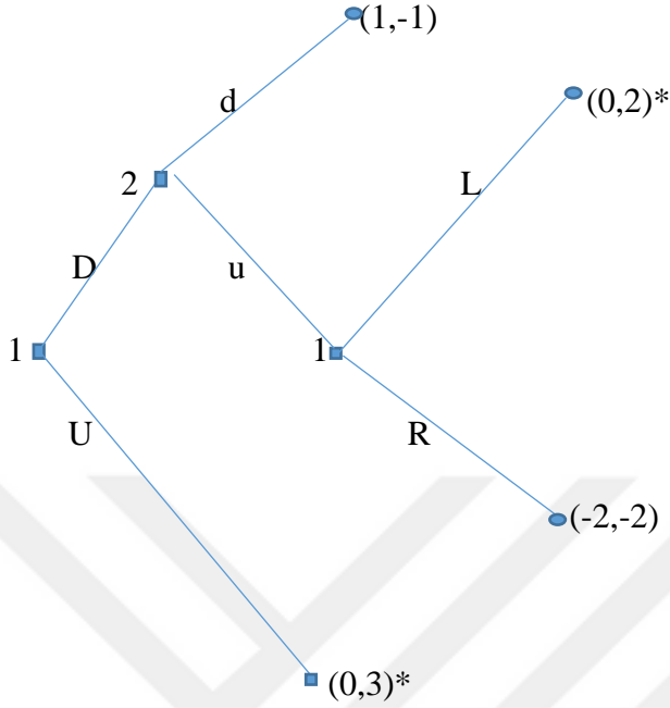
Şekil 9: Alt Oyun Mükemmel Denge 419
