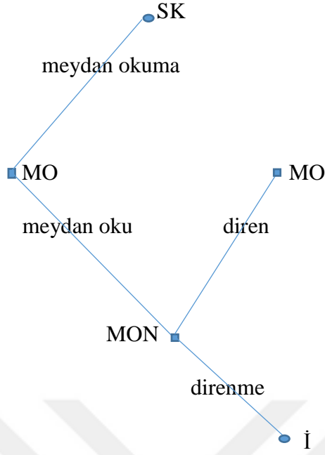
Şekil 3: Ağaç Gösterimi: Diren, Direnme 312
