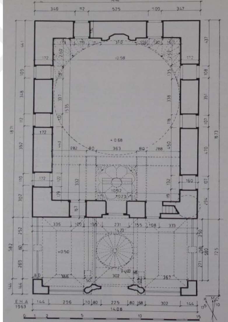
İznik Yeşil Cami planı (Ayverdi, Osmanlı Mimarisinin İlk Devri , I, 310)
