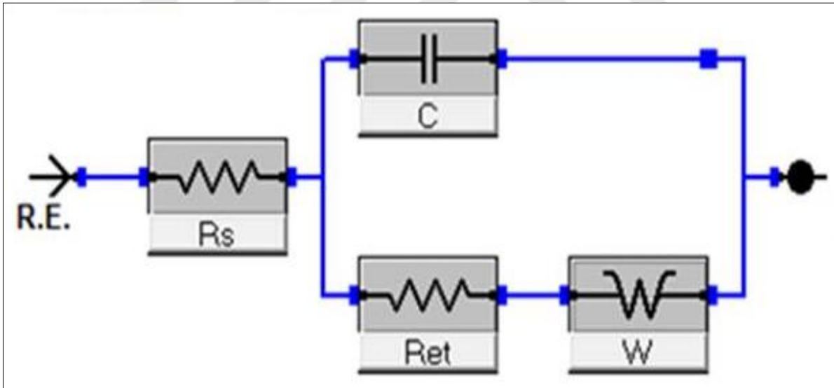
Şekil 3. 2. Biyosensör sisteminde kullanılan elektriksel eşdeğer devre modeli [ R_s : çözelti direnci, C : kapasitans, R_{et} : elektron transfer rezistansı, W : warburg impedansı] ( Karaboğa ve Sezgintürk 2018 )
