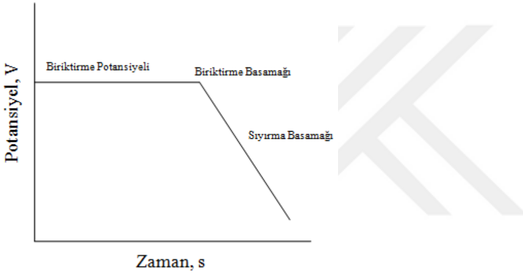
Şekil 2.4. Sıyırma yöntemlerinde zaman ile potansiyelin değişimi
