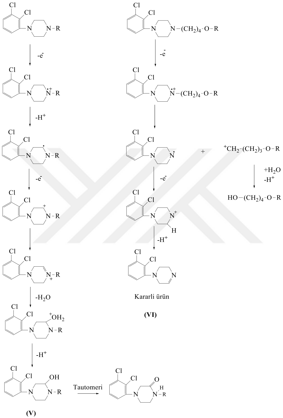
Şekil 4.12. ARP moleküllerinin Al 2 O 3 NP-KPE yüzeyinde gerçekleşen elektroyükseltgenme reaksiyonu için önerilen mekanizmalar
