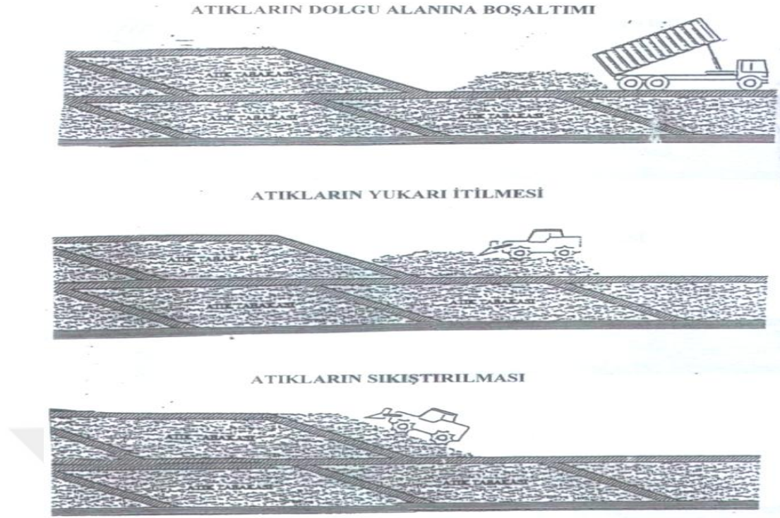
Şekil 4.15. Atık Tabakalarının Sıkıştırılarak Oluşturulması
