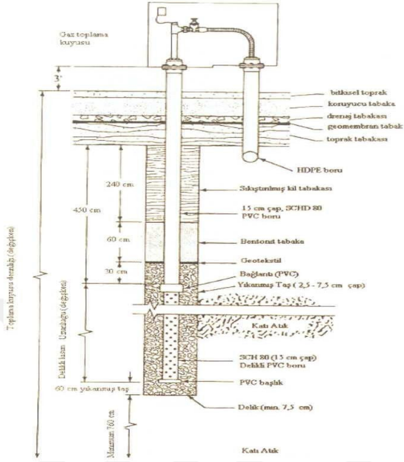
Şekil 2.15. Düşey Gaz Toplama Kuyusu ve Başlığı Detayları (Öztürk 2010).
