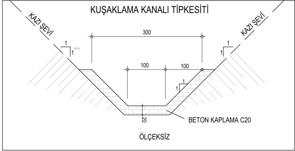
Şekil 4.14. Doğu-Güney Kanadı Kuşaklama Kanalı Tip Kesiti
