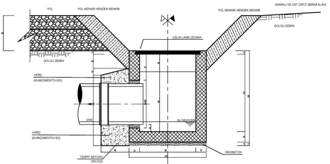
Şekil 4.11. Yağmur Suyu Su Alma Yapısı
