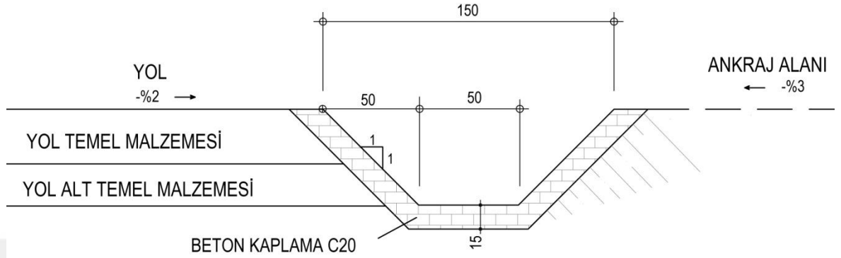
Şekil 4.10. Yol Kenarı Kanalı Tip Kesiti
