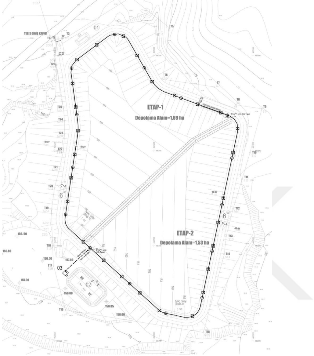
Şekil 4.20. Sızıntı Suyu Geri Devir Hattı Planı
