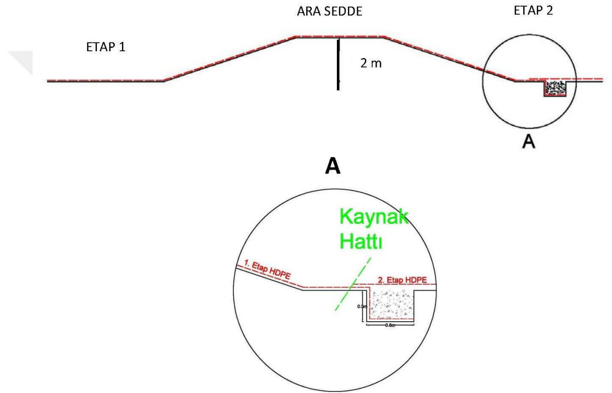
Şekil 4.8. Etap Ayırma Seddesi Tip Ankraj Kesiti
