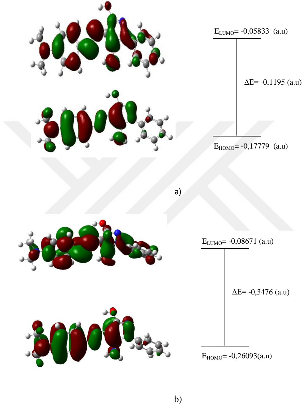
Şekil 5.11: B molekülünün a) DFT/B3LYP ve b) HF seviyeleri ile hesaplanmış HOMO-LUMO orbitalleri.
