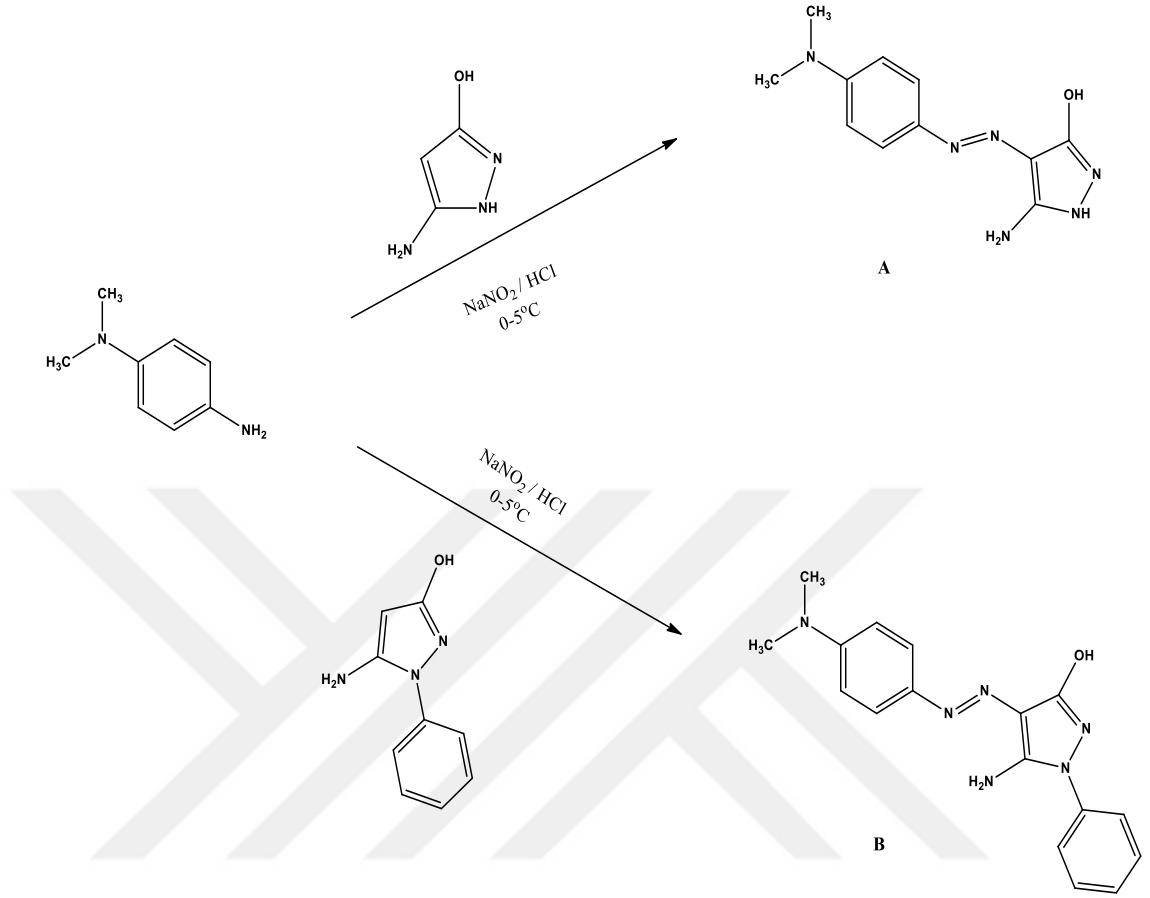
Şekil 4.1: A ve B moleküllerinin sentezlenme şeması.
