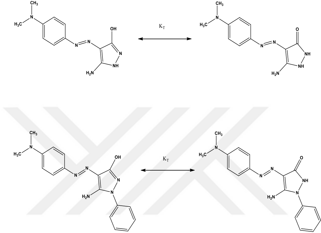
Şekil 4.2: A ve B bileşiklerinin totomerik yapıları.
