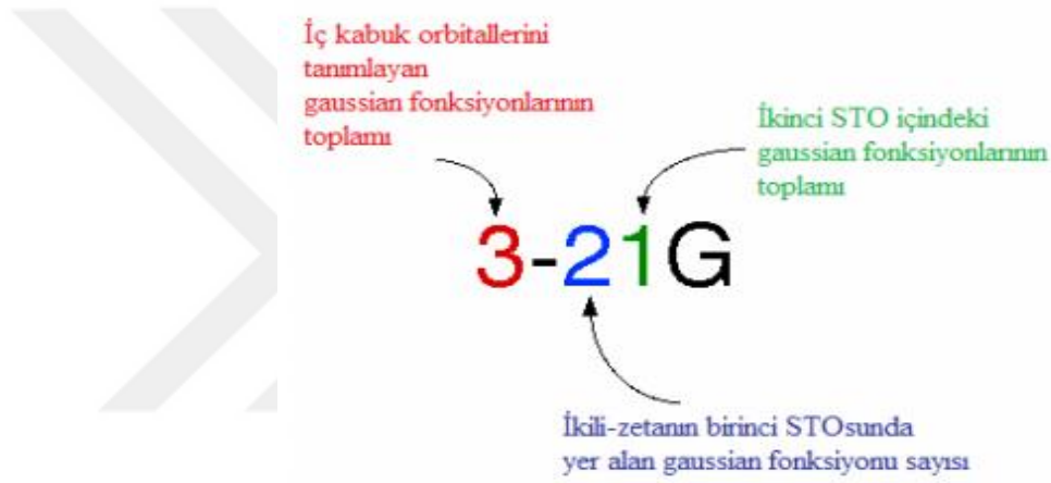
Şekil 3.1: Temel Setlerin Tanımlanması.
