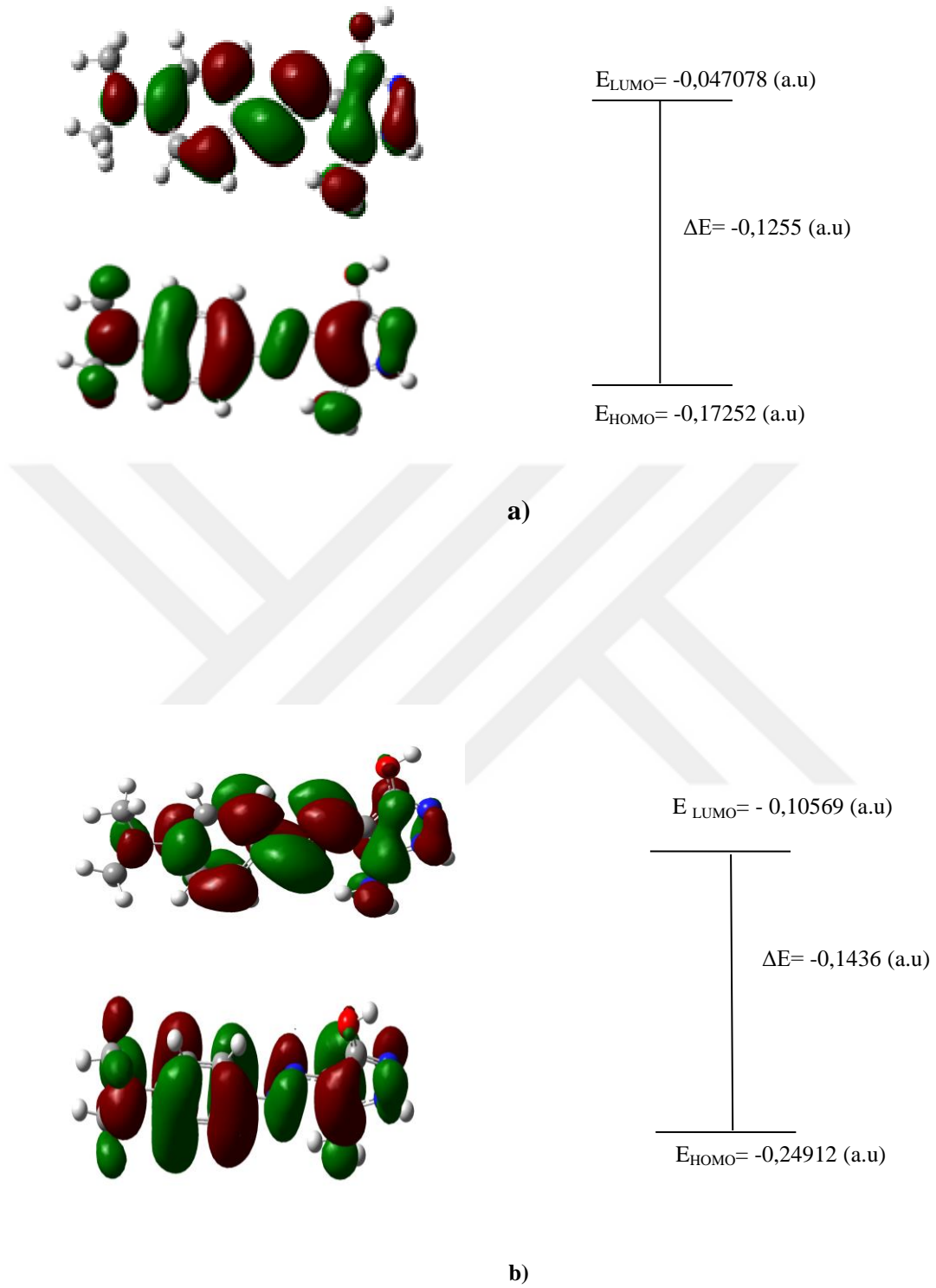
Şekil 5.10: A molekülünün a) DFT/B3LYP ve b) HF seviyeleri ile hesaplanmış HOMO-LUMO orbitalleri.
