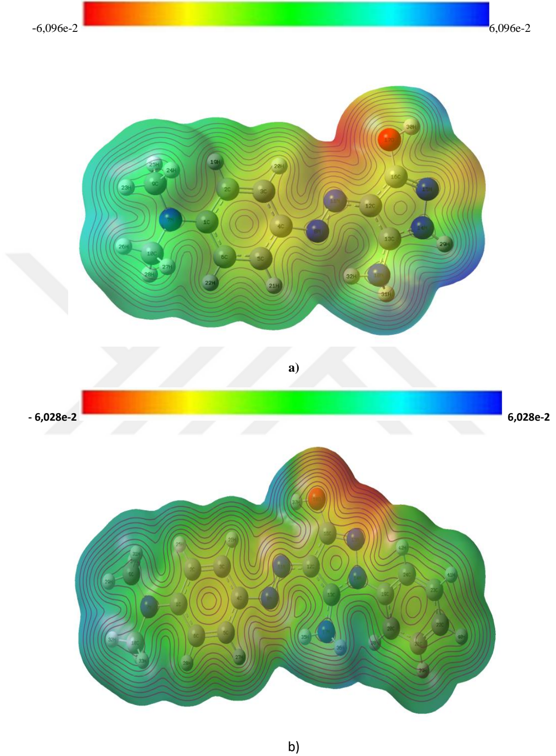
Şekil 5.12: a) A Molekülüne, b) B Molekülüne ait DFT/ B3LYP seviyesi ile hesaplanmış MEPs haritası.
